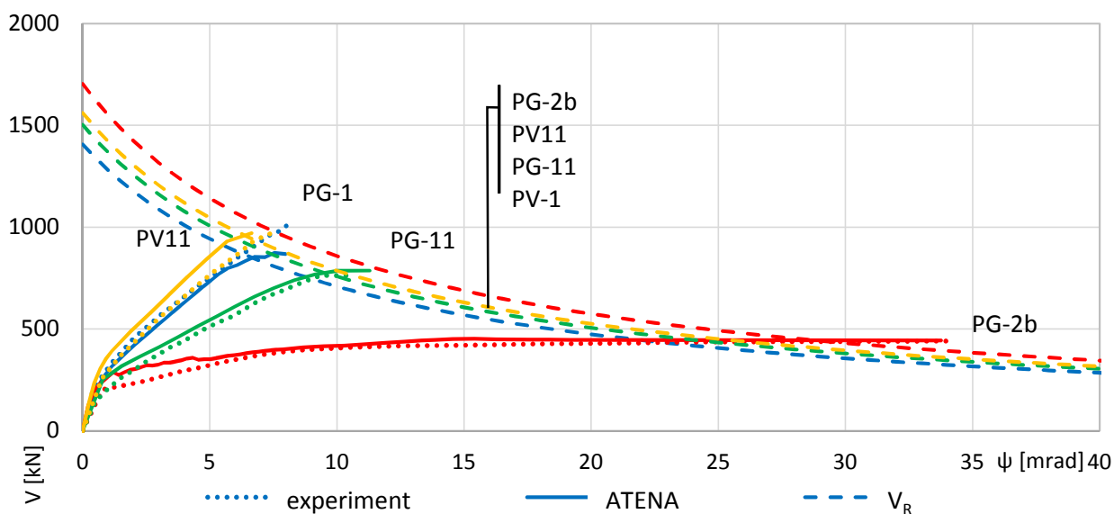
Obr. 9 Porovnání křivek zatížení – pootočení jednotlivých experimentů s analytickými modely a křivky selhání dle CSCT
