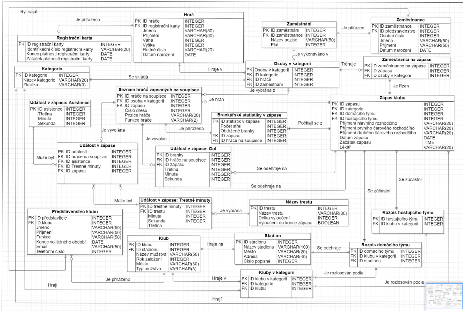
Obrázek 45 - Entity Relationship diagram, Zdroj: Vlastní zpracování
