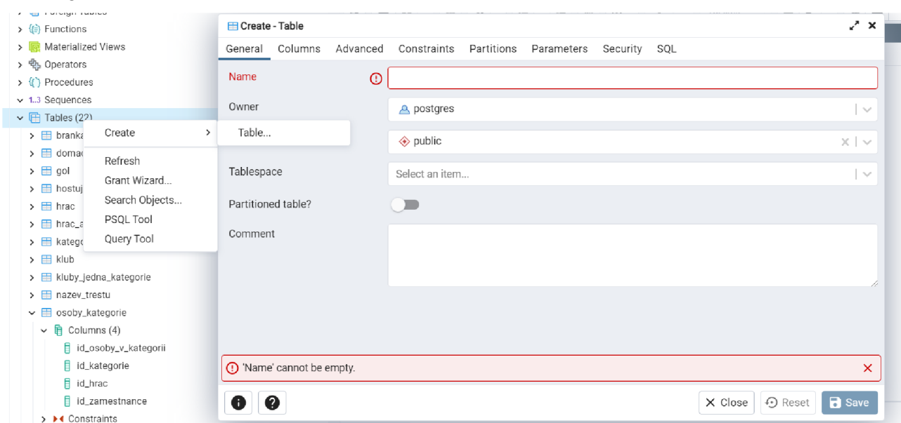
Obrázek 46- Vytvoření tabulky v PostgreSQL, Zdroj: Vlastní zpracování
