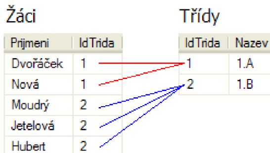
Obrázek 23-příklad SQL vztahu 1: více,Zdroj: (cdn.dotnetportal 2022)
