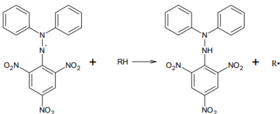
Obr. 4. Struktura DPPH a jeho redukce antioxidantem RH
