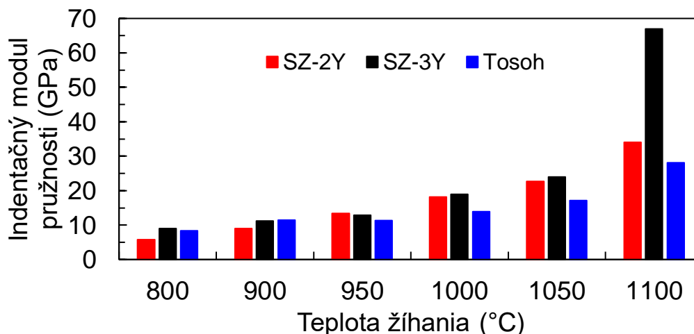
Obr. 5.3 Graf Indentačného modulu pružnosti vyžíhaných a obrobených telies v závislosti na teplote žihania.
