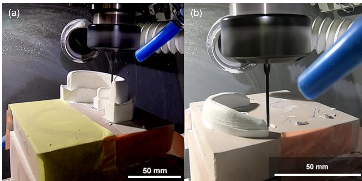
Obr. 5.28 Štádiá obrábania vyžihaneho tvarového polotovaru SZ-3Y 1000/1 pre čiastočnú náhradu kolenného kĺbu – (a) prvý krok, (b) druhý krok.
