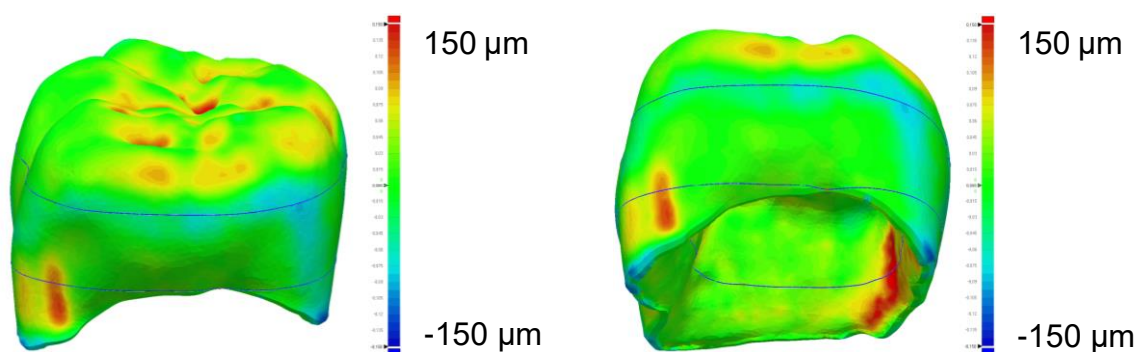
Obr. 5.30 Geometrické presnosť keramickej dentálnej korunky SZ-3Y 1550/2 – farebne škálovaná 3D mapa (a) horná časť; (b) spodná časť.
