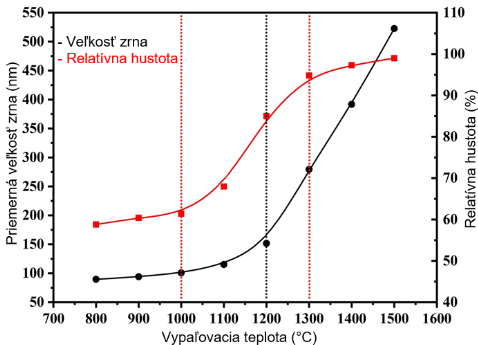
Obr. 2.6 Vplyv teploty na hodnotu relatívnej hustoty telesa a veľkosti zrna. [7]
