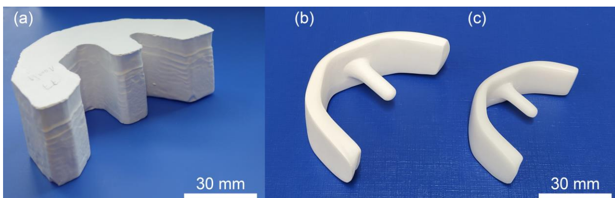
Obr. 5.29 Štádiá obrábania vyžihaneho tvarového polotovaru pre čiastočnú náhradu kolenného kĺbu – (a) tvarový polotovar SZ-3Y 1000/1, (b) obrobené teleso SZ-3Y 1000/1 a (c) vypálené teleso SZ-3Y 1550/2.
