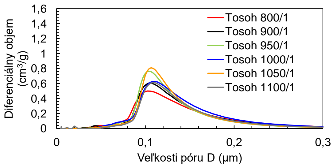
Príloha 1 Distribúcia veľkosti pórov žíhaných vzoriek.
