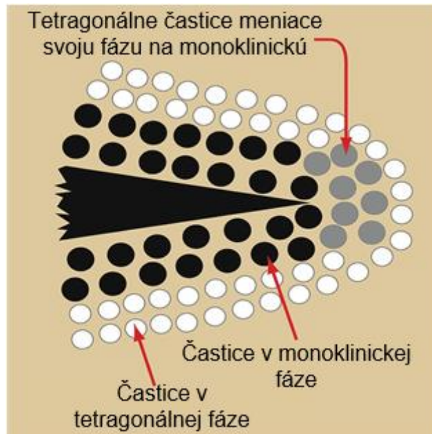
Obr. 2.2 Proces spevňovania materiálu fázovou transformáciou. [10]
