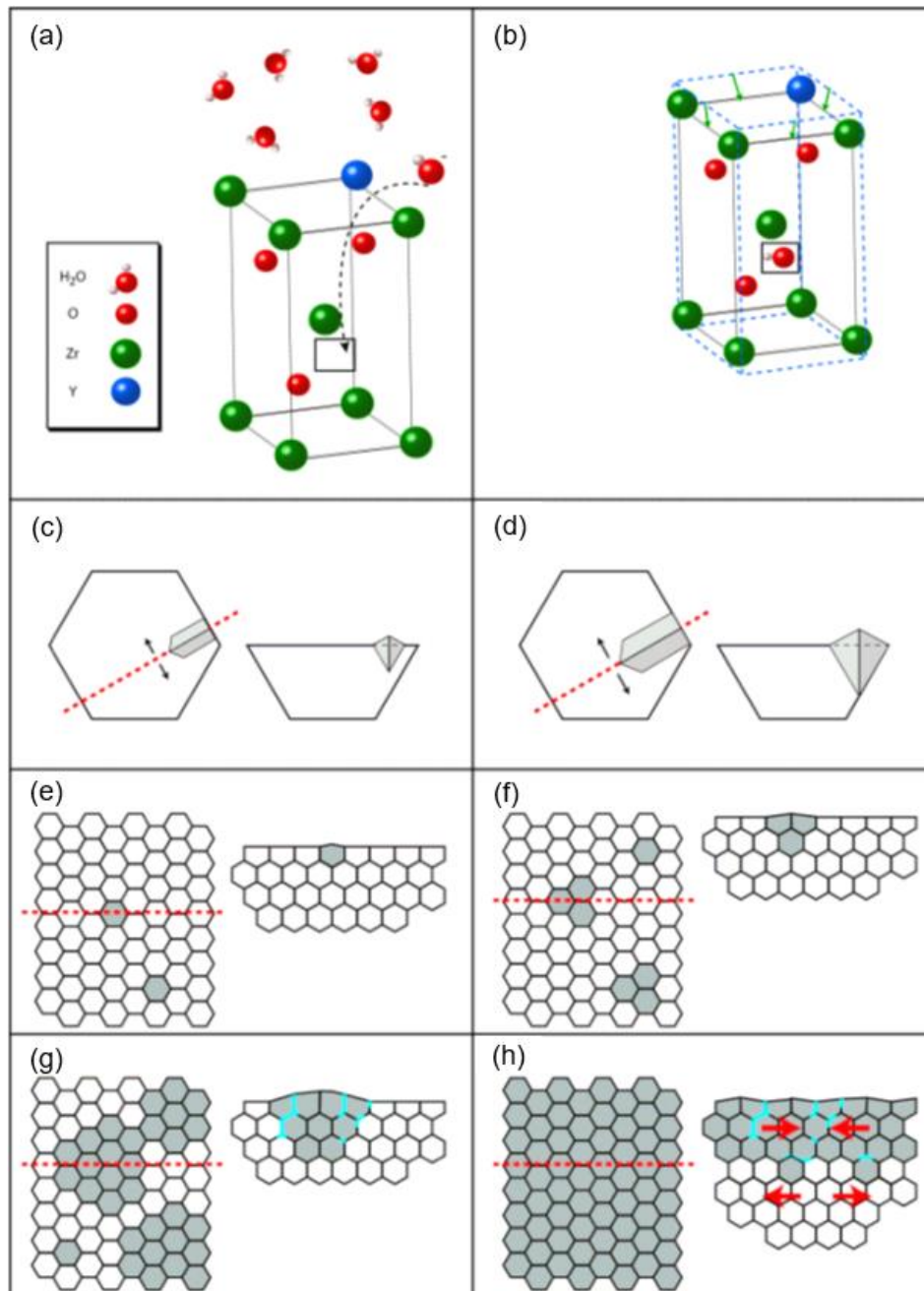
Obr. 2.11 Priebeh procesu LTD. [14]
