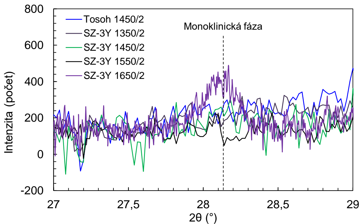
Obr. 5.16 Detail oblasti s charakteristickým vrcholom monoklinickej fázy pre vzorky s 3 mol. % Y_2O_3 .
