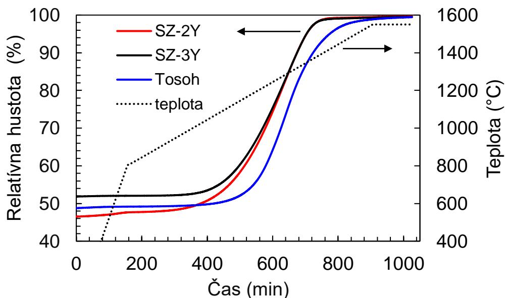
Obr. 5.12 Graf závislosti relatívnej hustoty na čase pri ohreve a výdrži 2h na teplote 1550 °C.
