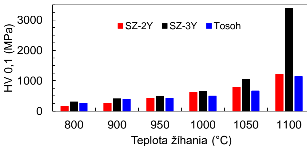
Obr. 5.2 Graf tvrdosti vyžíhaných a obrobených telies v závislosti na teplote žihania.
