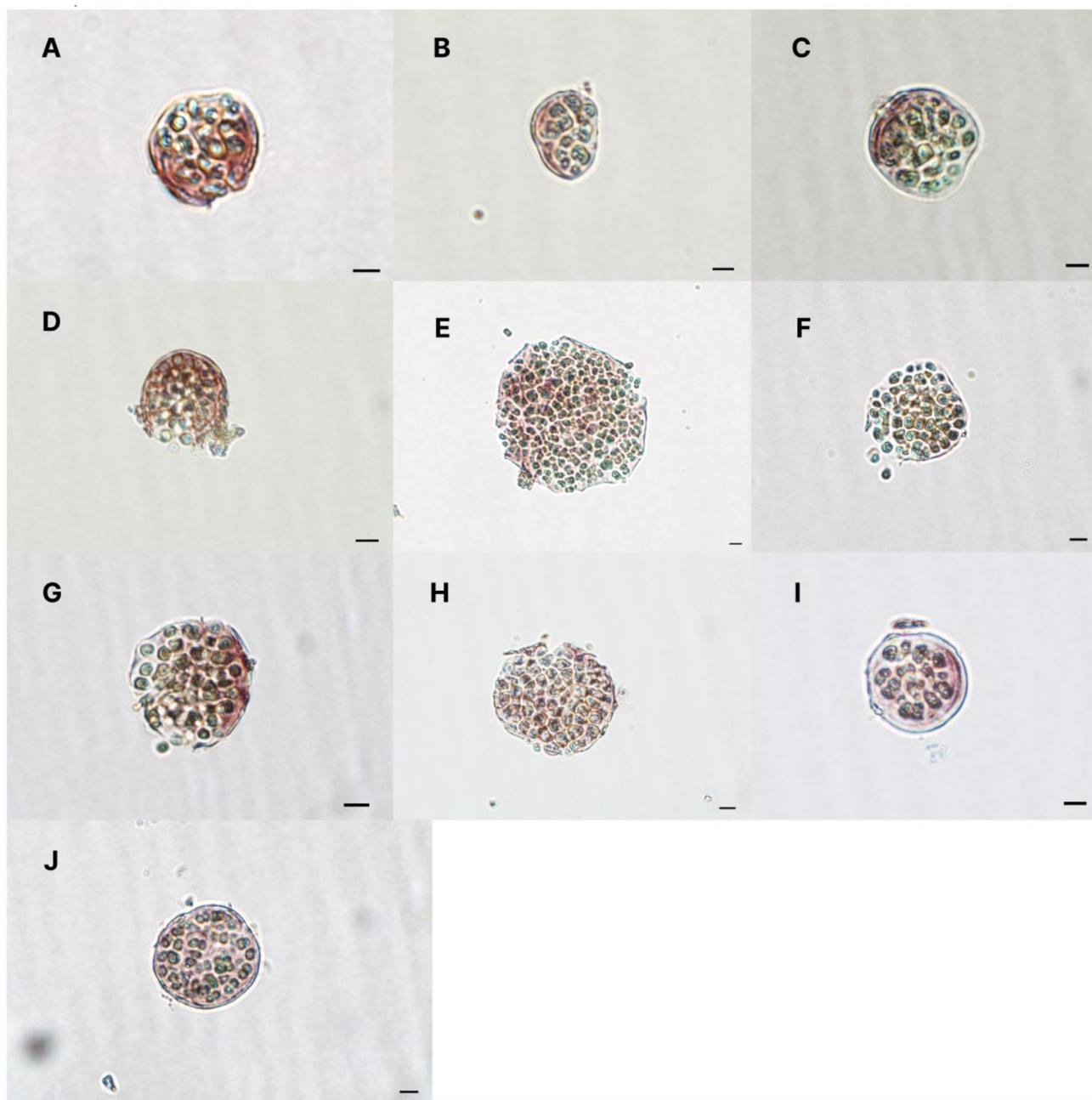
Obrázek 7. Izolované kolonie Gloeocapsa violascea ze vzorku č. 8 (Opolenec). Světle fialová barva odpovídá pH pufru (7,2). A- vzorek 8.1; B- vzorek 8.2; C- vzorek 8.3; D- vzorek 8.4; E- vzorek 8.6; F- vzorek 8.7; G- vzorek 8.8; H- vzorek 8.9, I- vzorek 8.10, J- vzorek 8.11. Měřítko = 10 \mu\text{m} .
