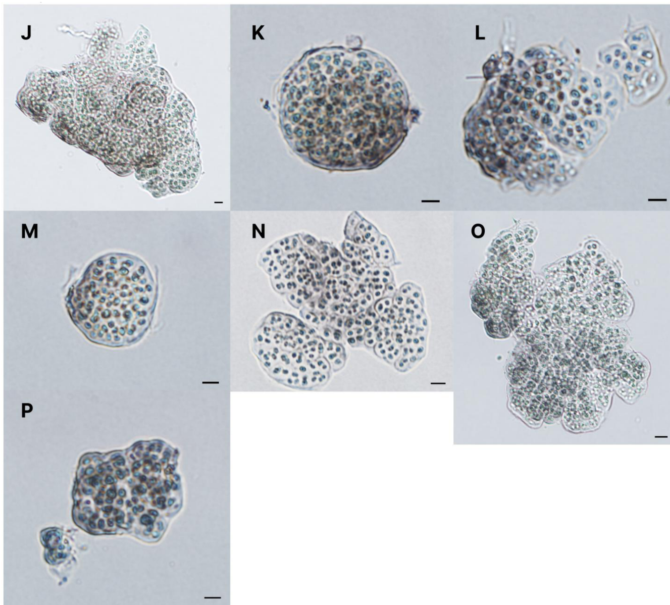
Obrázek 8b. Izolované kolonie Gloeocapsa atrata ze vzorku č. 20 (Holubovské hadce). Světle fialový odstín odpovídá pH pufru (7,2). J - vzorek 20.10, K - vzorek 20.11, L - vzorek 20.12, M - vzorek 20.13, N - vzorek 20.14, O - vzorek 20.15, P - vzorek 20.16. Měřítko = 10 \mu\text{m} .
