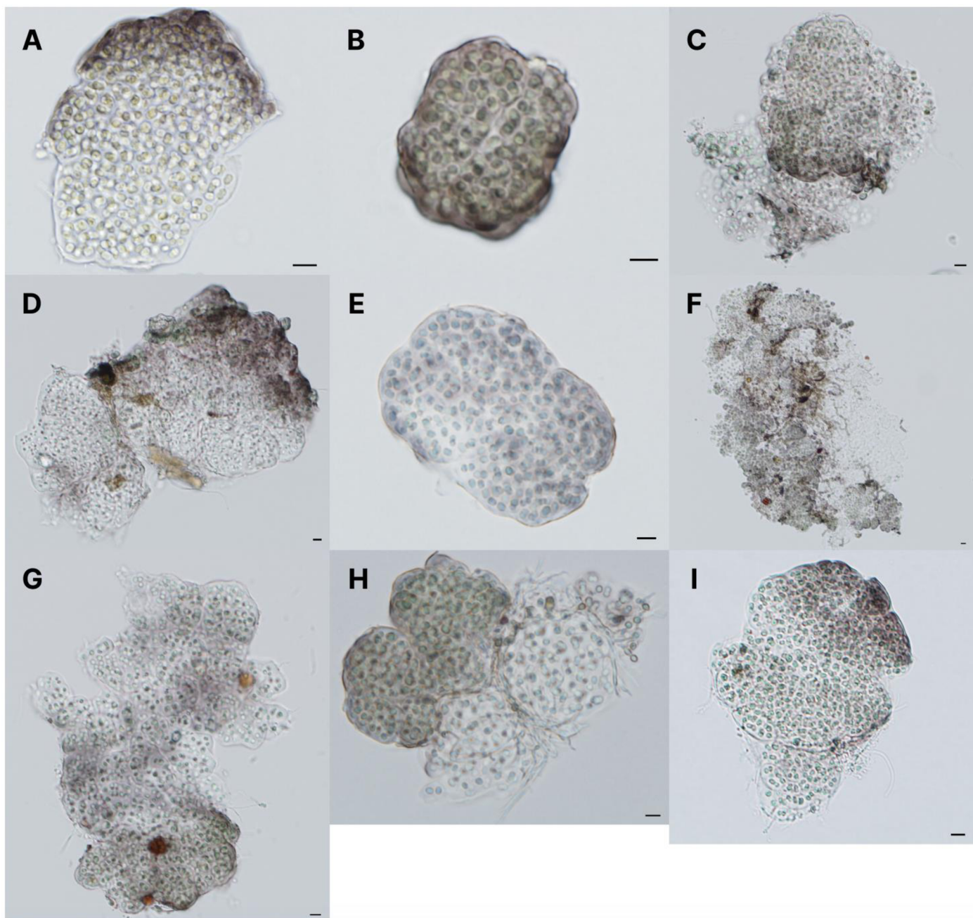
Obrázek 8a. Izolované kolonie Gloeocapsa atrata ze vzorku č. 20 (Holubovské hadce). Světle fialový odstín odpovídá pH pufru (7,2). A- vzorek 20.1; B- vzorek 20.2; C- vzorek 20.3; D- vzorek 20.4; E- vzorek 20.5; F- vzorek 20.6; G- vzorek 20.7; H- vzorek 20.8, I- vzorek 20.9. Měřítko = 10 \mu\text{m} .
