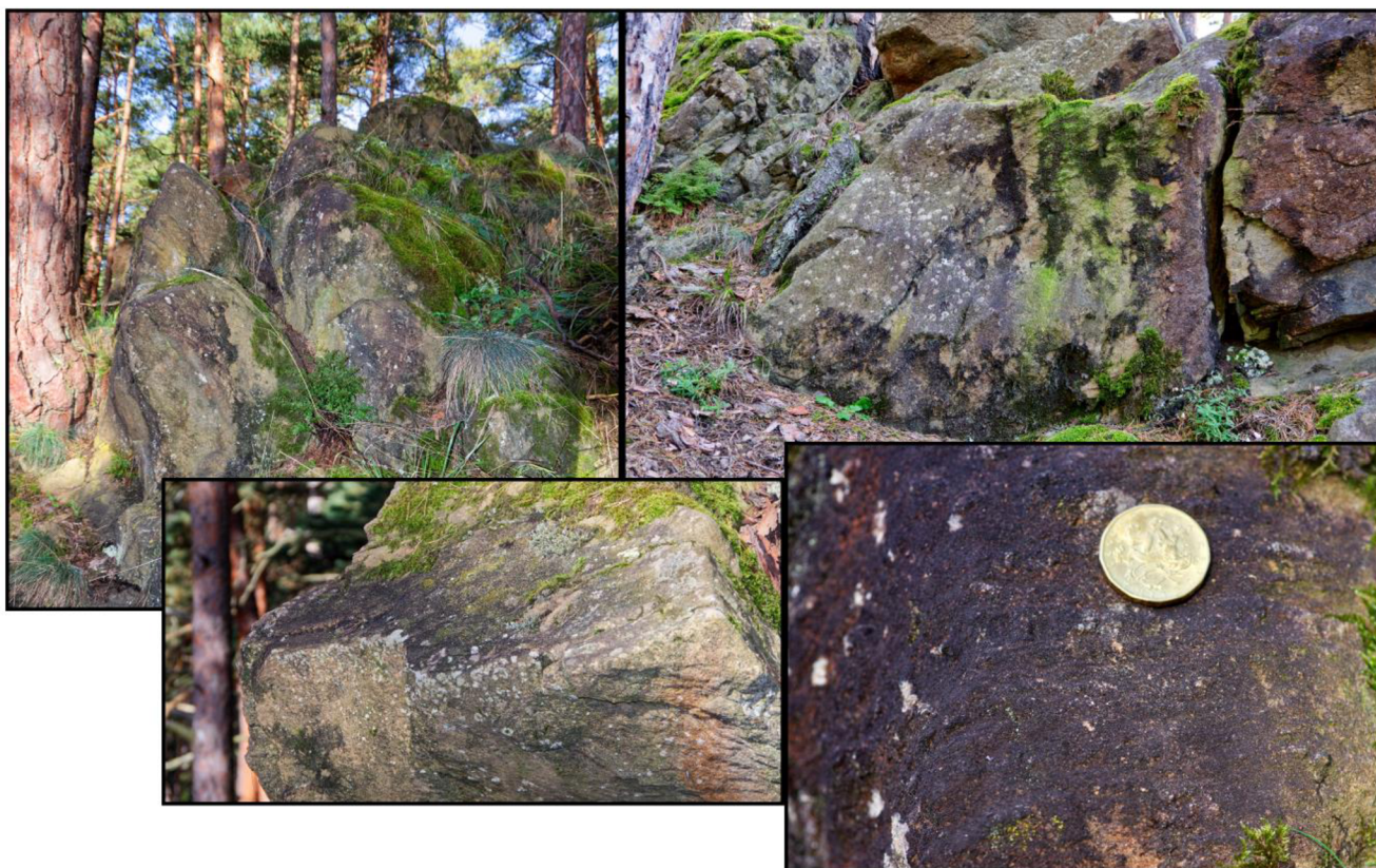
Obrázek 4. Holubovské hadce, epilittické nárosty sinic.
