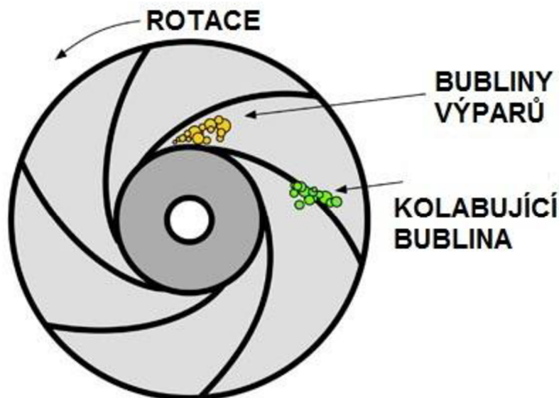
Obr. 3.6 Kavitace hydrodynamického čerpadla [30]
