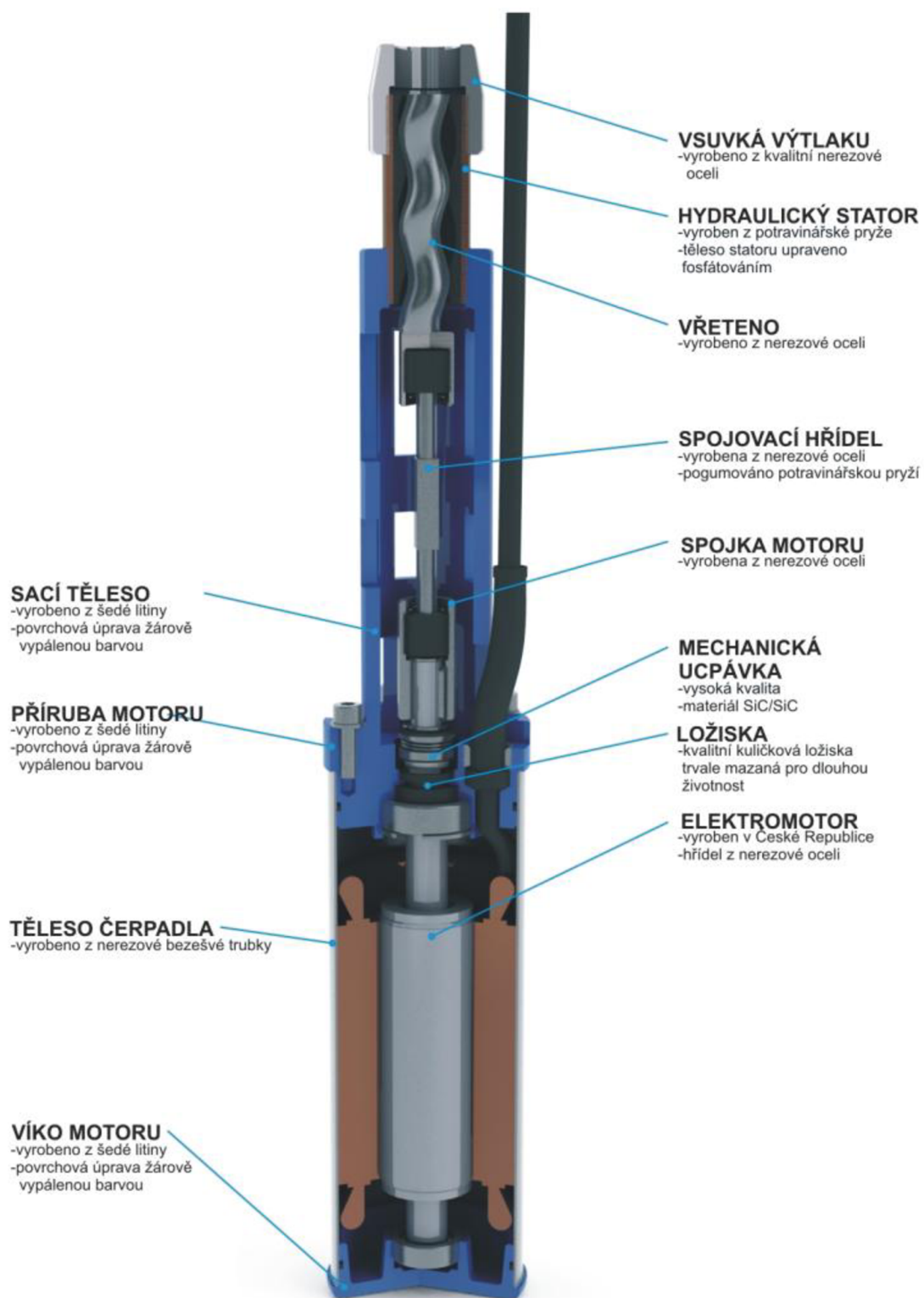
Obr. 3.7 Řez hydrostatického ponorného vřetenového čerpadla [15]
