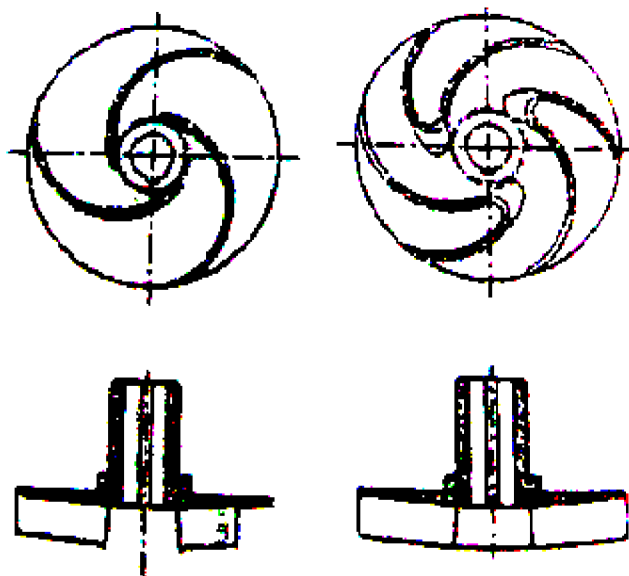
Obr. 3.1 Vícekanalová oběžná kola používaná při čerpání odpadních vod [12]
