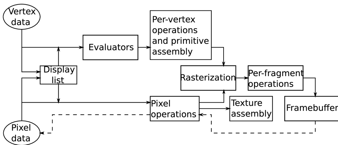
Obrázek 3.3: Vykreslovací řetězec
