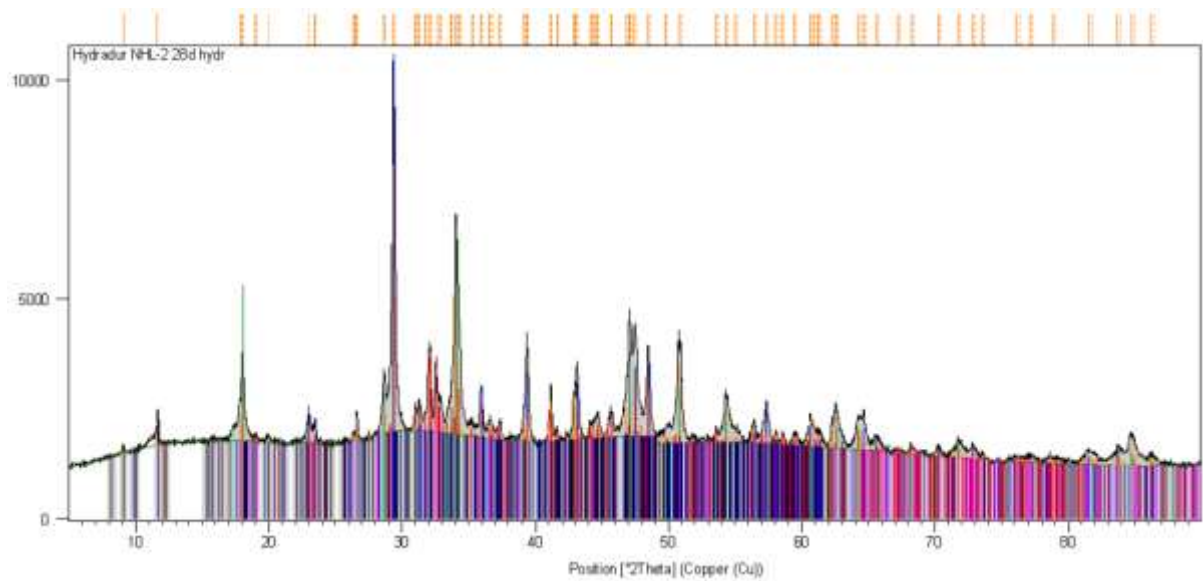
Obrázok 27: Záznam z röntgenovej analýzy vzorky Calcidur NHL-2 po 28 dňoch od hydratácie.
