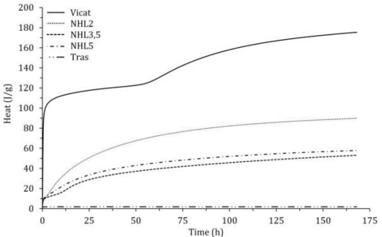
Obrázok 12: Tok tepla pri hydratácii vzoriek v [J/g] v závislosti od času.
