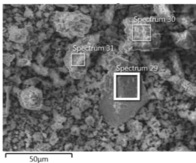
Obrázok 5: Záber zo SEM mikroskopie pre Calcidur NHL-2.
