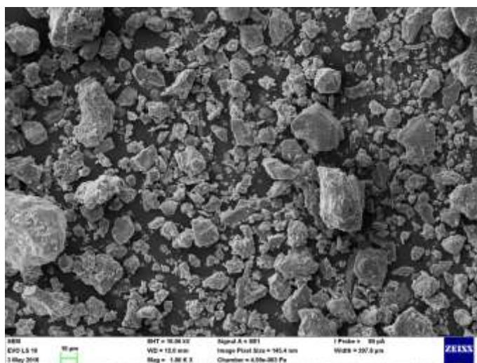
Obrázok 25: Snímok hydratovaného produktu vzorky Tras v zväčšení 1000 x po 28 dňoch od hydratácie.
