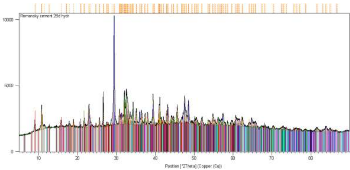
Obrázok 35: Záznam z röntgenovej analýzy vzorky Románsky cement po 28 dňoch od hydratácie.
