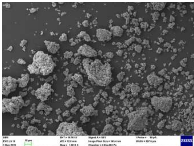
Obrázok 24: Snímok hydratovaného produktu vzorky Hydradur NHL-5 v zväčšení 1000 x po 28 dňoch od hydratácie.
