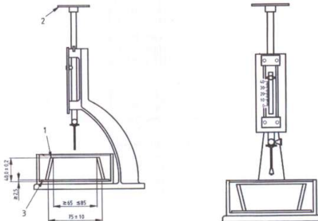
Obrázok 2: Stanovenie počiatku a konca tuhnutia na Vicatovom prístroji 1 – prstenec, 2 – plocha na prídavné závažie, 3 – podložná doštička [12]
