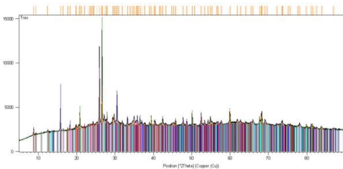
Obrázok 31: Záznam z röntgenovej analýzy vzorky Tras.
