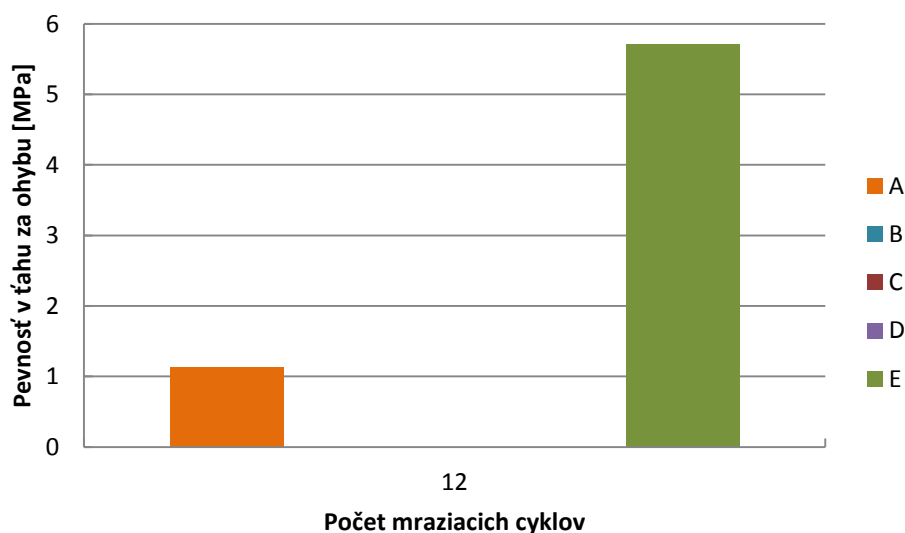
Obrázok 18: Pevnosť v tahu za ohybu vzoriek uskladnených vo vrečku po 12 mraziacich cykloch. A – Calcidur NHL-2, B – Calcidur NHL-3,5, C – Hydradur NHL-5, D – Tras, E – Románsky cement.
