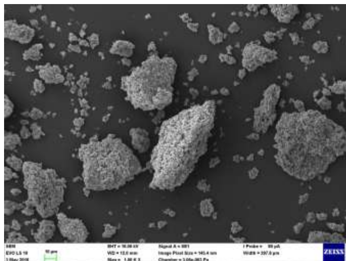
Obrázok 23: Snímok hydratovaného produktu vzorky Calcidur NHL-3,5 v zväčšení 1000 x po 28 dňoch od hydratácie.
