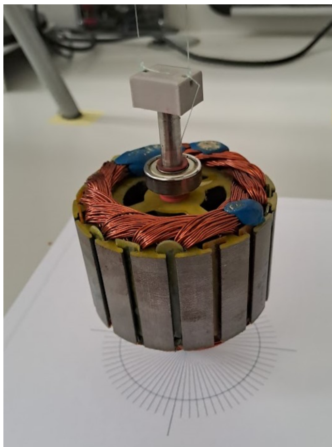
Obrázek 3.19: Zavěšení rotoru
