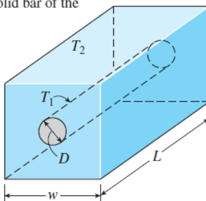
Obrázek 3.16: Tvarový součinitel vedení [7]
