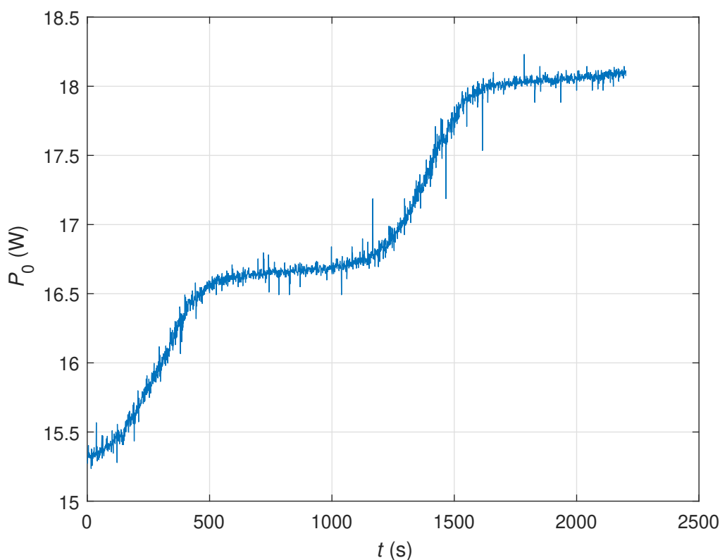
Obrázek 3.14: Příkon do soustavy pro I = 8 A
