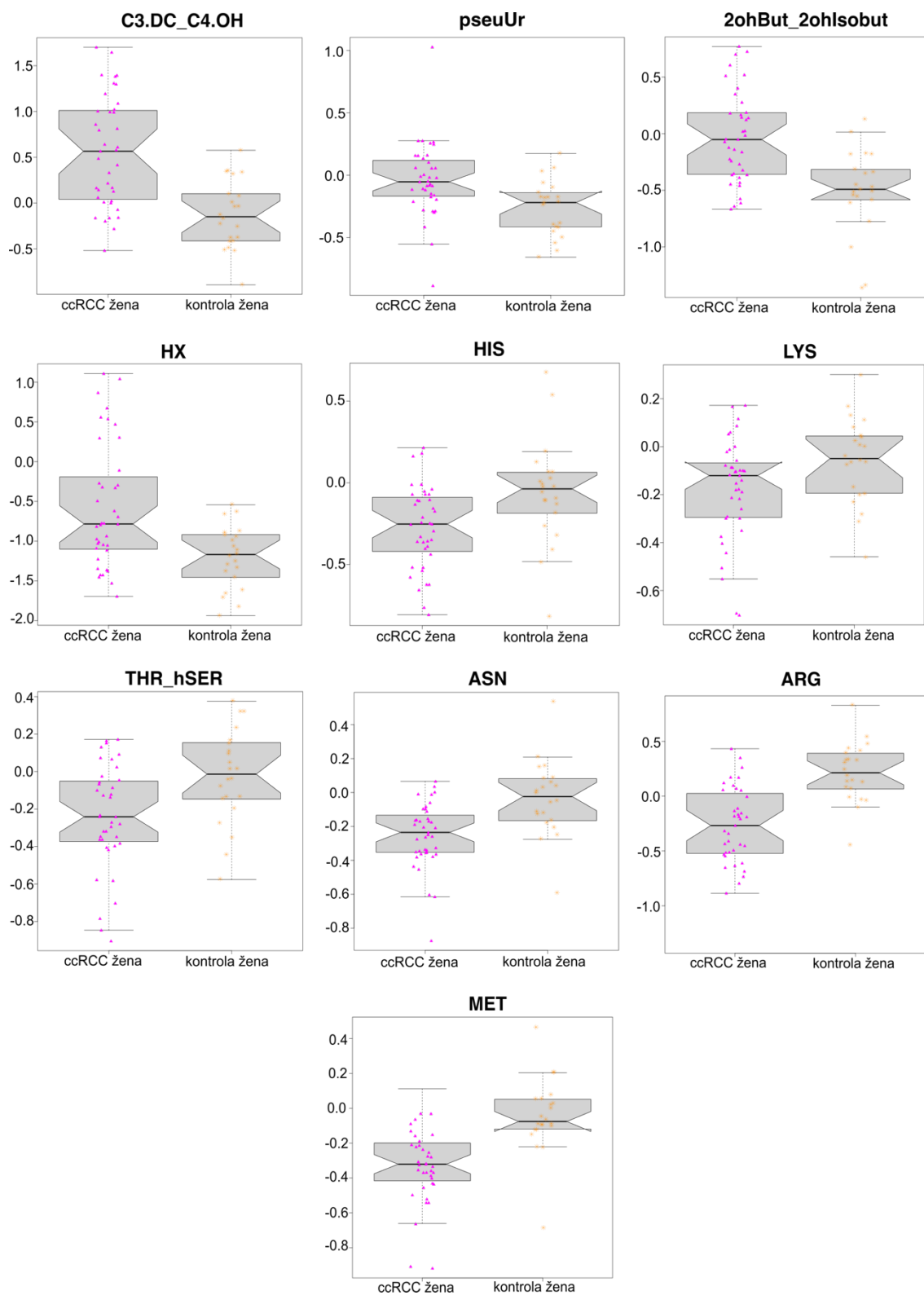
Obr. 23: Krabicové grafy zobrazujúci zvýšené/snížené hladiny významných metabolitů pro vícerozměrnou i jednorozměrnou statistickou analýzu u pacientek ženského pohlaví ve srovnání s kontrolami.
