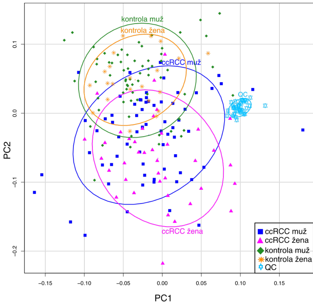
Obr. 15: PLS-DA analýza vzorků plazem od pacientů s ccRCC a kontrolních vzorků. Každý bod představuje jeden konkrétní vzorek ze skupin muži s ccRCC (tmavě modrá), ženy s ccRCC (růžová), kontrolní vzorky mužů (zelená), kontrolní vzorky žen (oranžová) a QC vzorky jsou vyznačeny světle modře.
