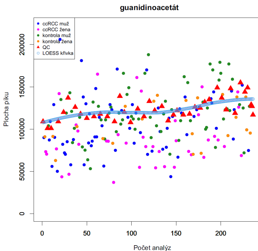
Obr. 13 Ilustrační obrázek interpolace guanidinoacetátu po aplikaci LOESS křivky.
