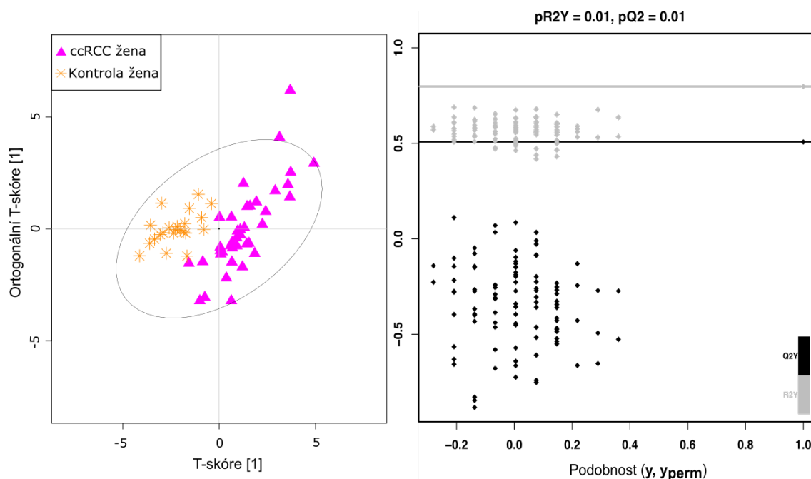
Ob. 17: Skórový graf metody OPLS-DA zobrazující oddělení vzorků do skupin ženy s ccRCC (růžové body) a kontrolní vzorky žen (oranžové body) s příslušným permutačním testem.
