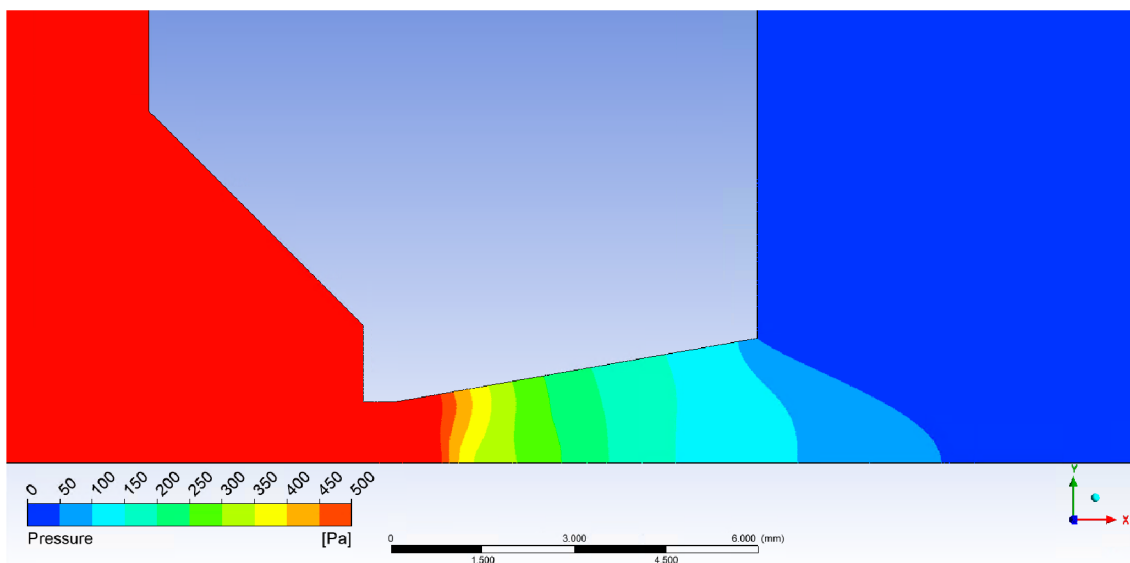
Obrázek 48 Varianta rozevření dýzy 10^\circ
