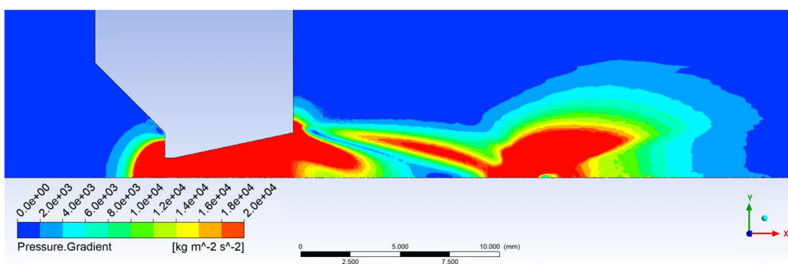
Obrázek 106 Varianta rozevření dýzy 12°
