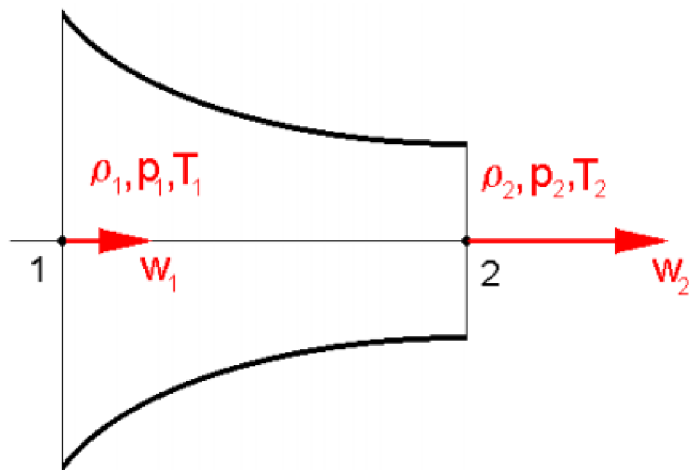
Obrázek 9 Kritický tlakový poměr
