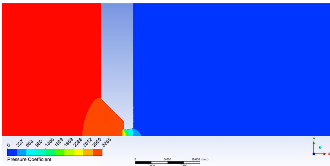
Obrázek 91 Varianta rozevření zkrácené dýzy 12^\circ
