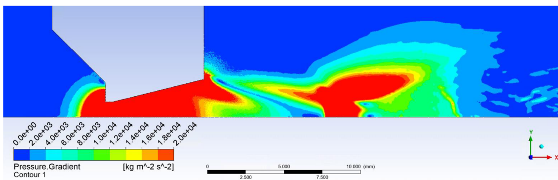
Obrázek 107 Varianta rozevření dýzy 14°
