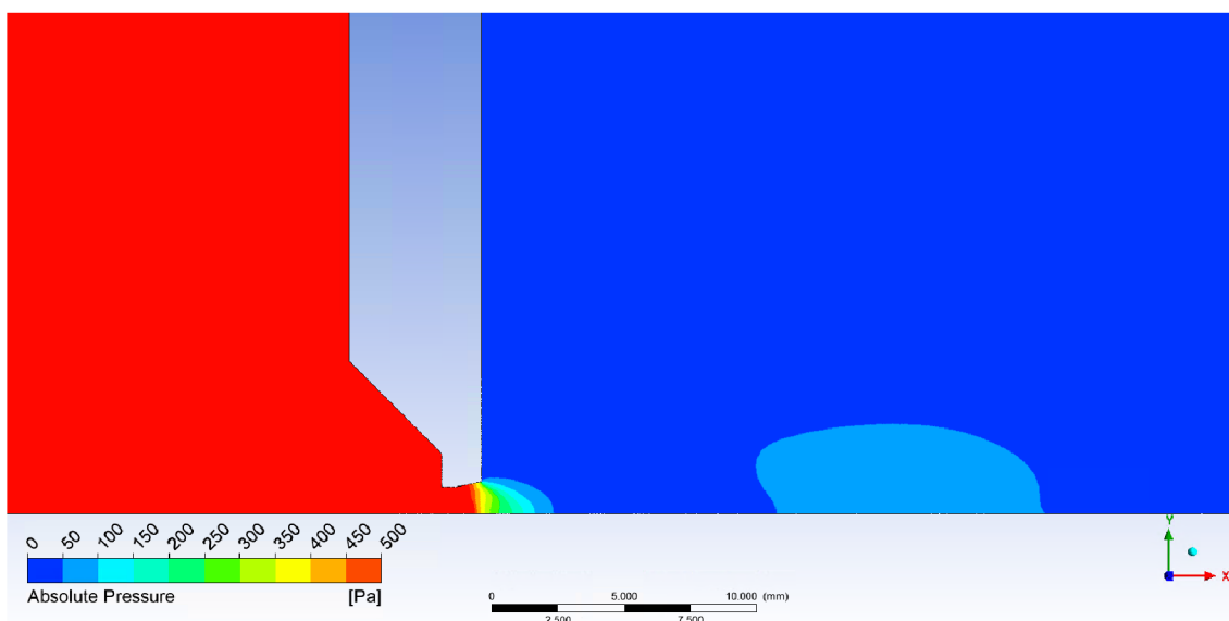
Obrázek 49 Varianta rozložení zkrácené dýzy 12^\circ
