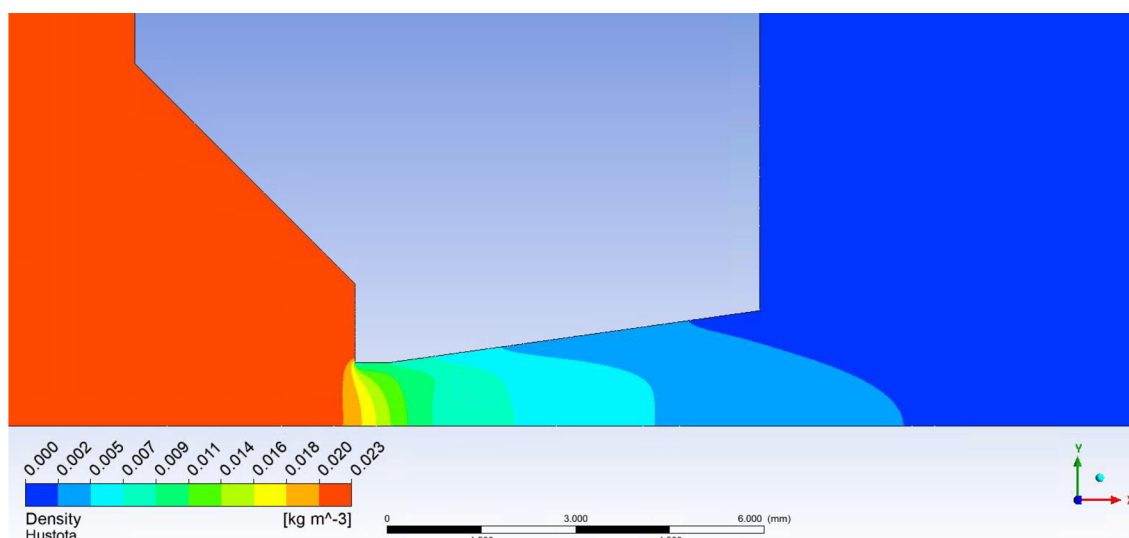
Obrázek 32 Rozložení hustoty pro variantu rozevření dýzy 8^\circ
