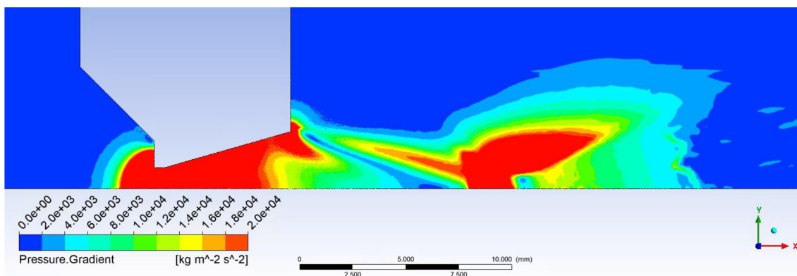
Obrázek 108 Varianta rozevření dýzy 16°
