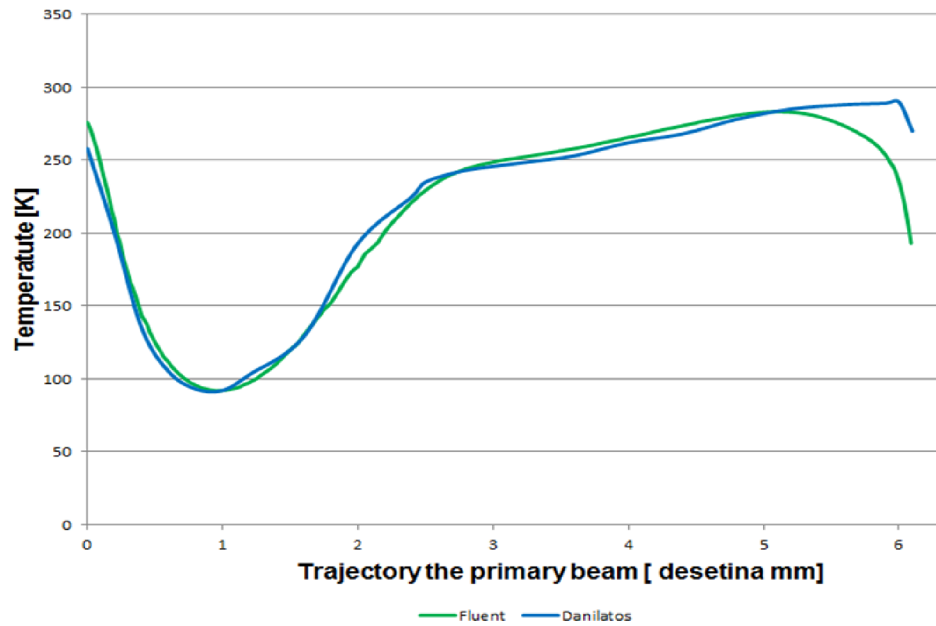
Obrázek 6 Srovnání výsledků simulace teploty obou metod
