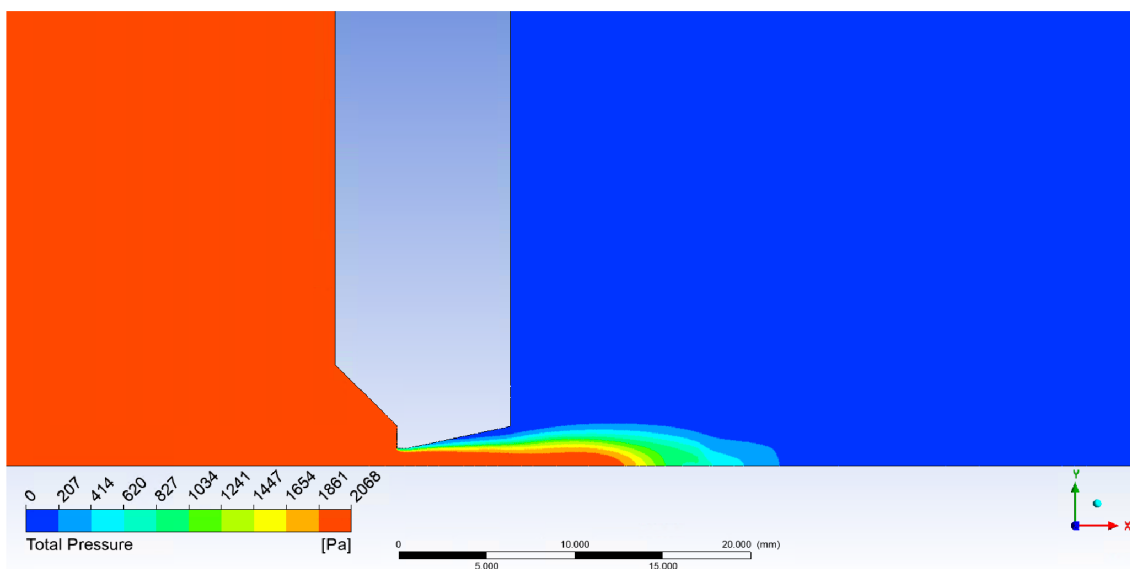
Obrázek 85 Varianta rozevření dýzy 12°
