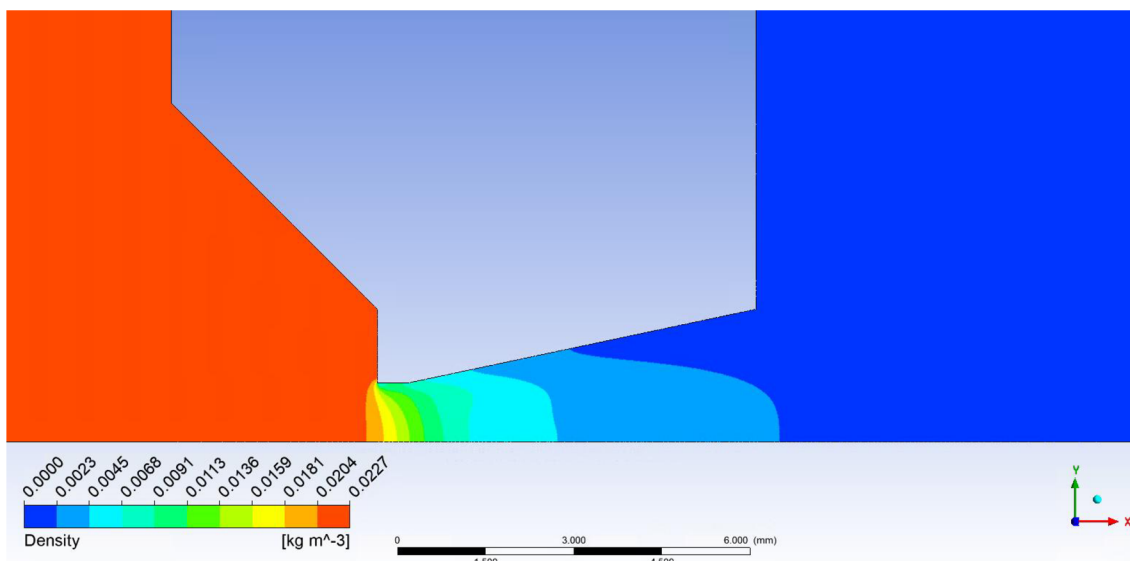
Obrázek 33 Rozložení hustoty pro variantu rozevření dýzy 12°
