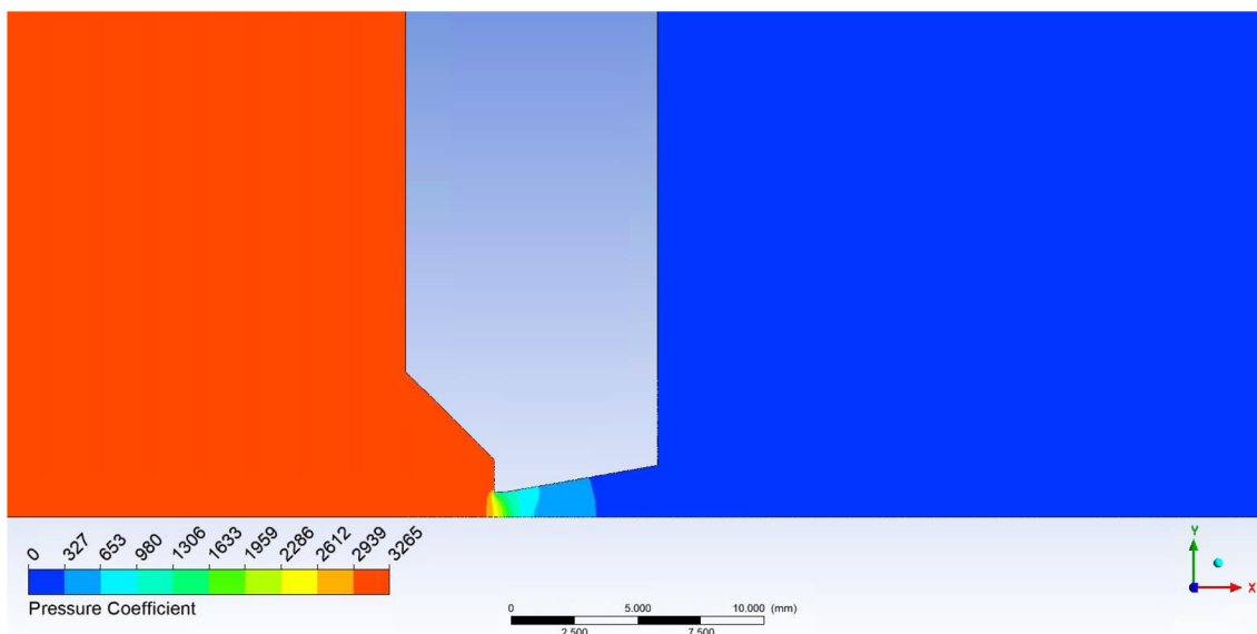
Obrázek 90 Varianta rozevření dýzy 10^\circ
