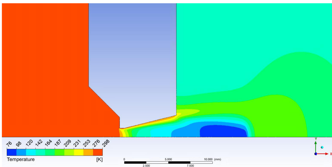
Obrázek 79 Varianta rozevření dýzy 14^\circ
