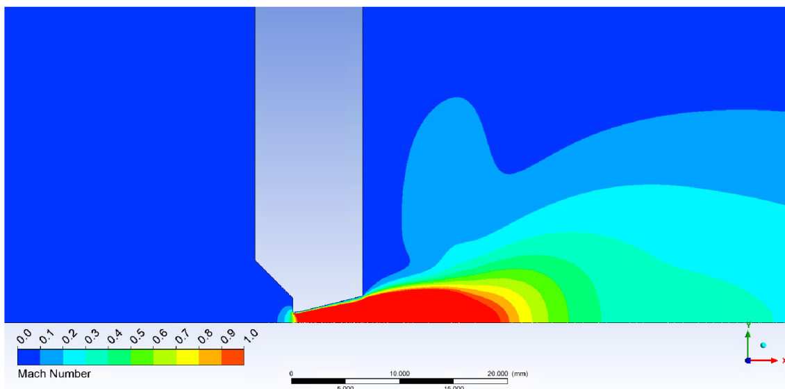
Obrázek 63 Varianta rozevření dýzy 14^\circ
