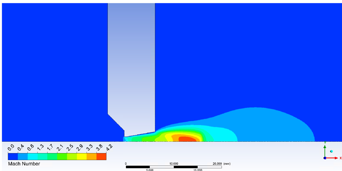
Obrázek 56 Varianta rozevření dýzy 10^\circ
