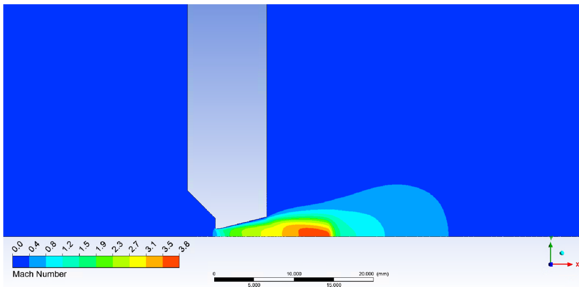
Obrázek 62 Varianta rozevření dýzy 14^\circ
