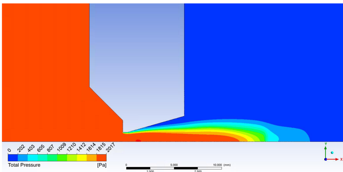
Obrázek 87 Varianta rozevření dýzy 16°
