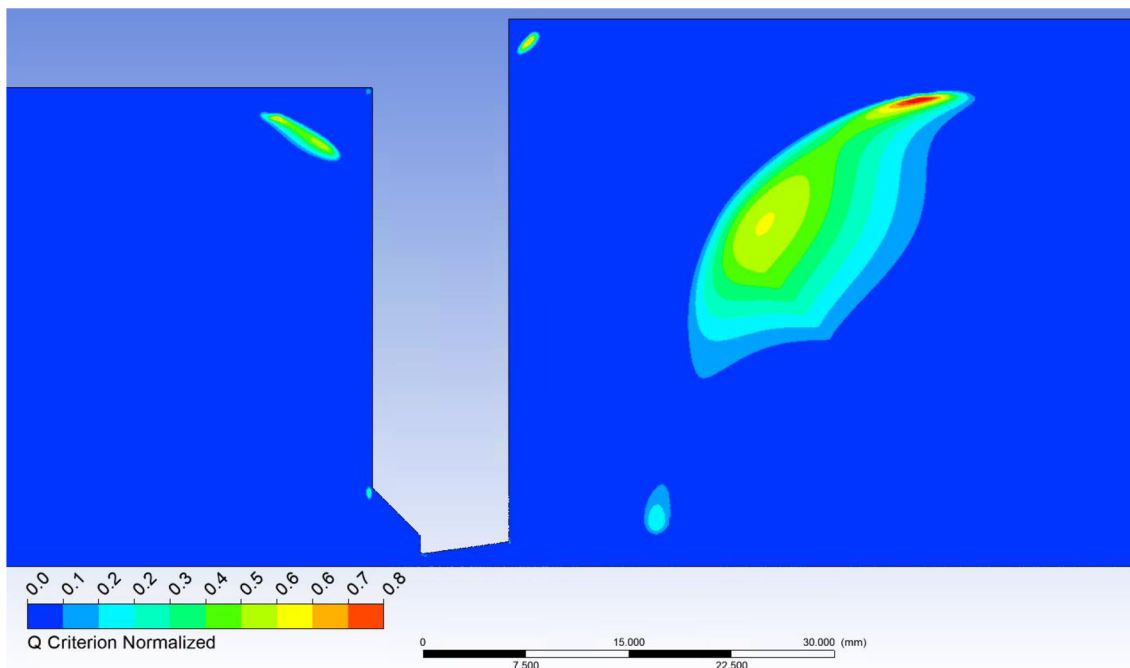
Obrázek 96 Varianta rozevření dýzy 8^\circ
