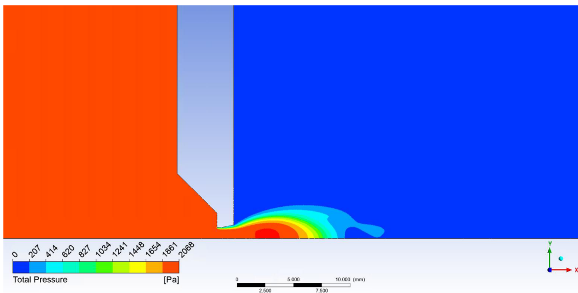
Obrázek 84 Varianta rozevření zkrácené dýzy 12°
