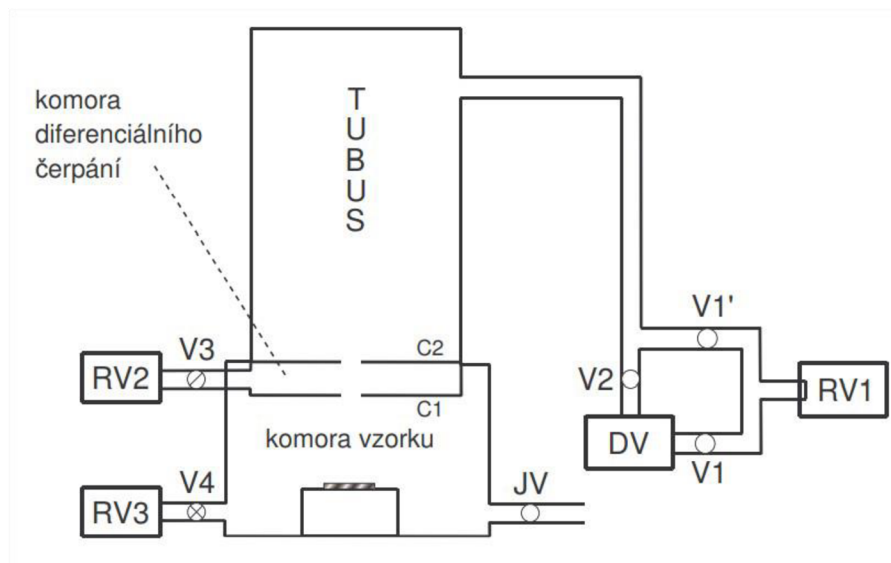
Obrázek 4 Vakuový systém environmentálního elektronového mikroskopu
