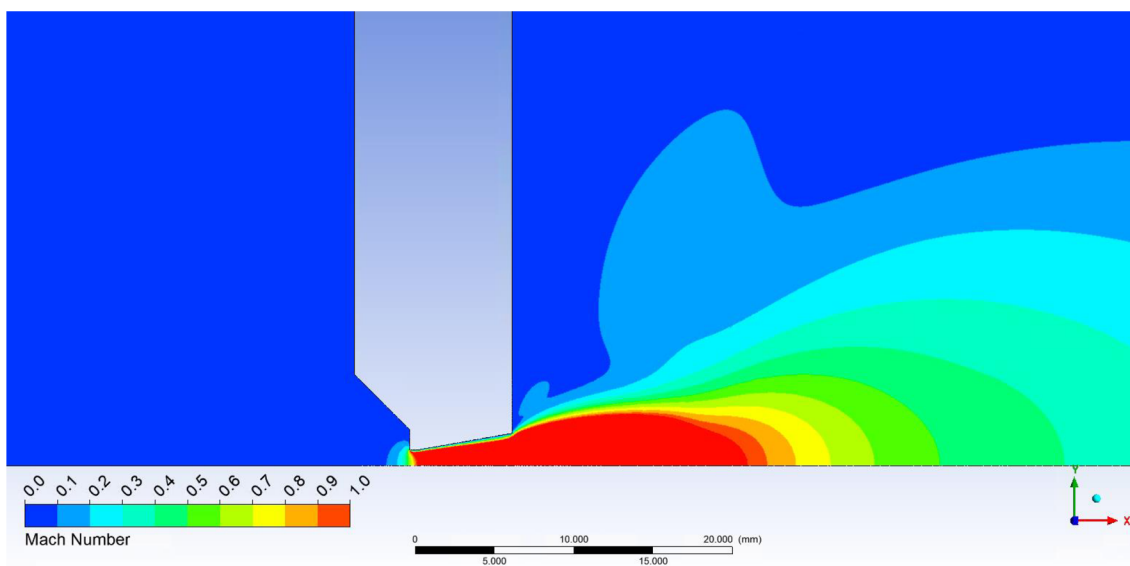
Obrázek 57 Varianta rozevření dýzy 10^\circ
