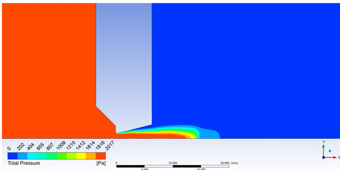
Obrázek 86 Varianta rozevření dýzy 14°
