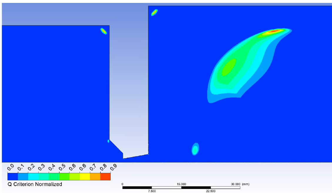
Obrázek 97 Varianta rozevření dýzy 10^\circ
