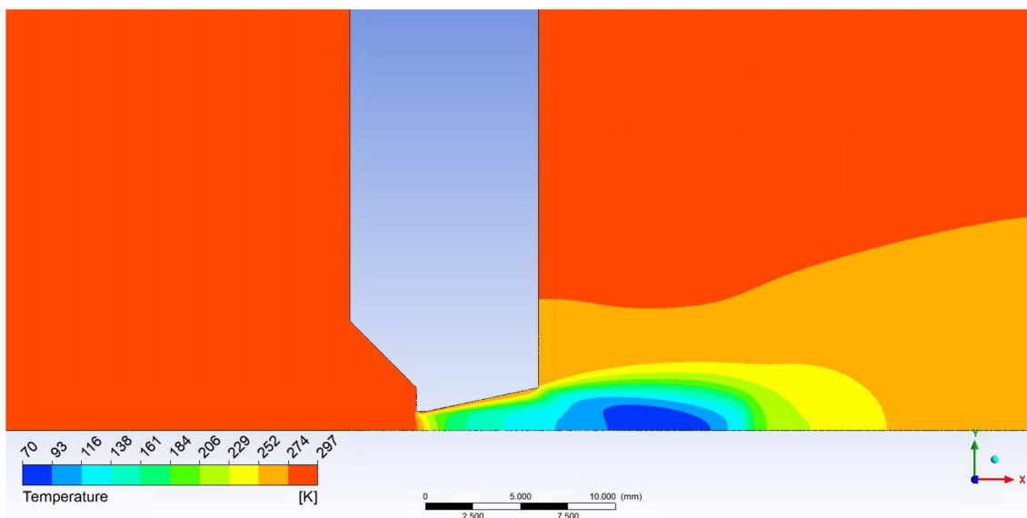
Obrázek 78 Varianta rozevření dýzy 12^\circ
