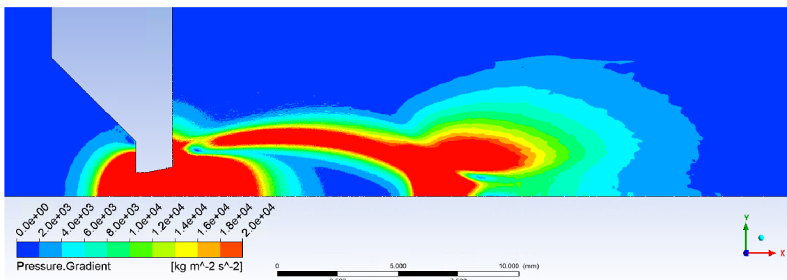
Obrázek 105 Varianta rozevření zkrácené dýzy 12°
