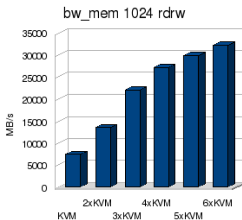
Obrázek 5.12: Propustnost paměti
