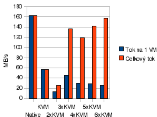
Obrázek 5.13: Prostupnost blokového čtení z disku
