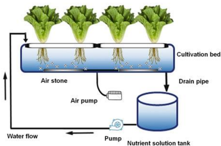
Obrázek 2.2: Schéma metody DFT (Kozai, 2018)
