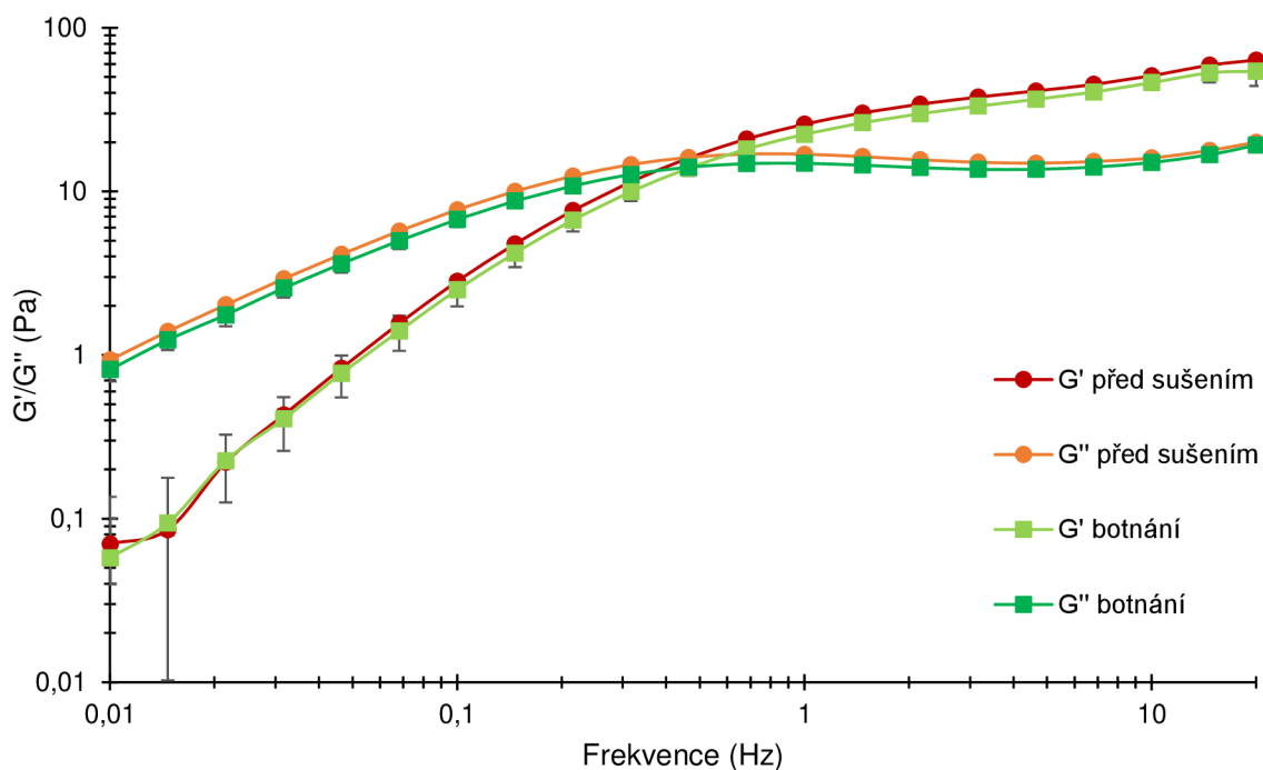
Obrázek 34: Závislost viskózního ( G'' ) a elastického ( G' ) modulu na frekvenci pro ověření schopnosti botnáni
