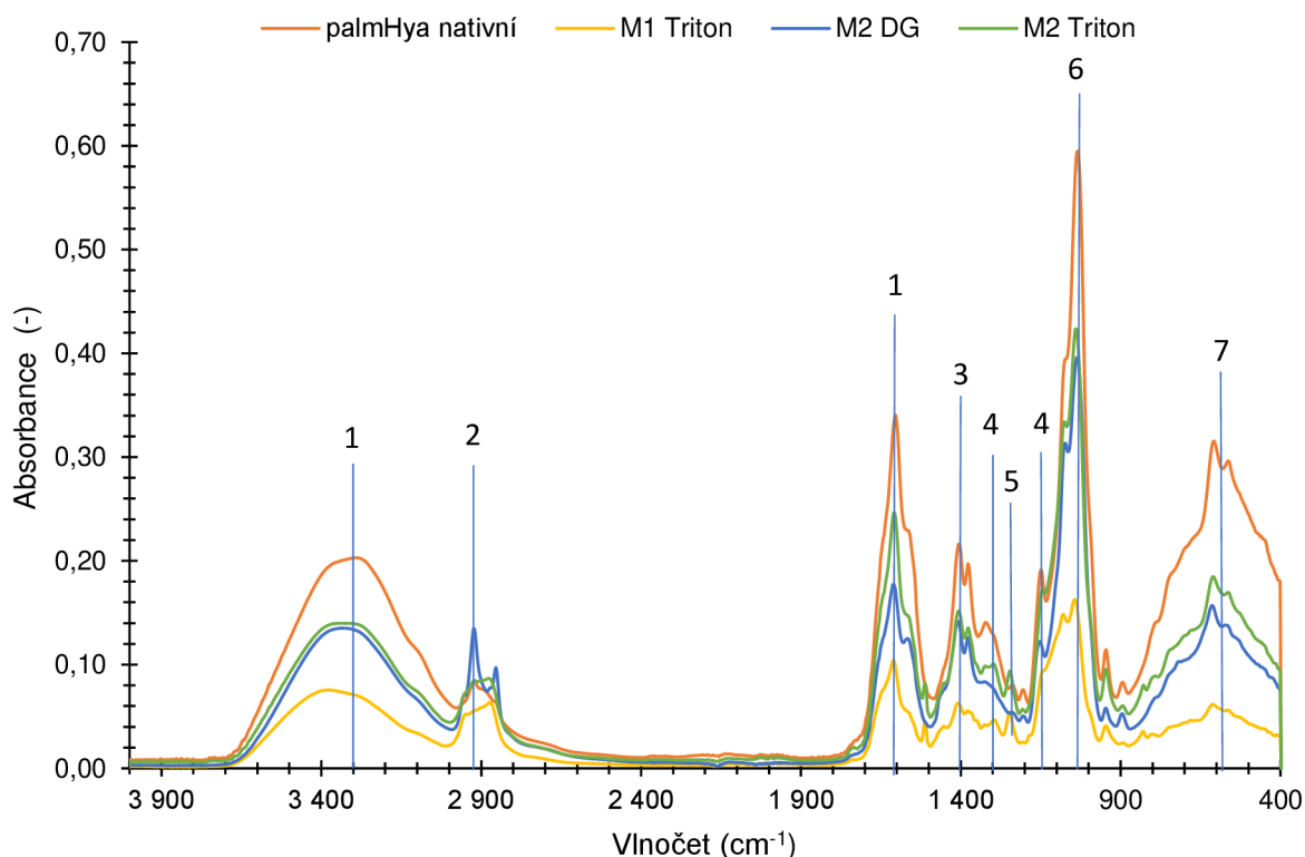
Obrázek 29: FT-IR spektra pro vysušené vzorky připravených hydrogelů
