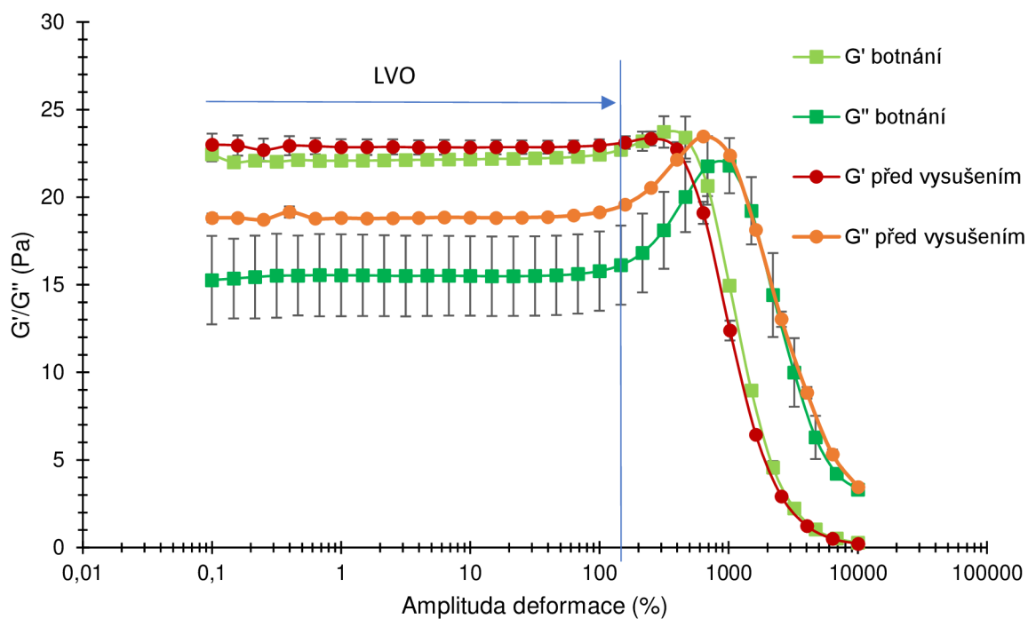
Obrázek 33: Závislost viskózního ( G'' ) a elastického ( G' ) modulu na amplitudě deformace pro ověření schopnosti botnáni
