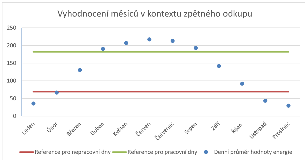
Obr. 18 Vizualizace průběhu výkonu v typický slunný den ve vztahu k průměrně spotřebované elektrické energii v pracovní a nepracovní den pro konkrétní měsíce
