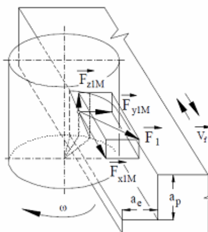
Obr. 4.7 Fyzikální model zatížení řezného nástroje v průběhu obrábění 4
