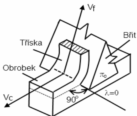
Obr. 2.9 Ortogonální řezání 5,7
