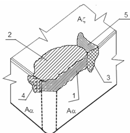
Obr.3.2 Formy opotřebení bříty 5
