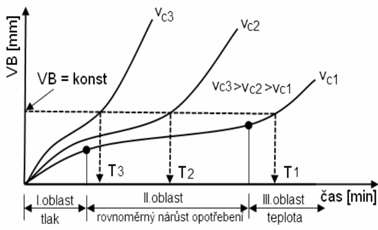
Obr.3.4 Časová závislost opotřebení pro různé řezné rychlosti 5
