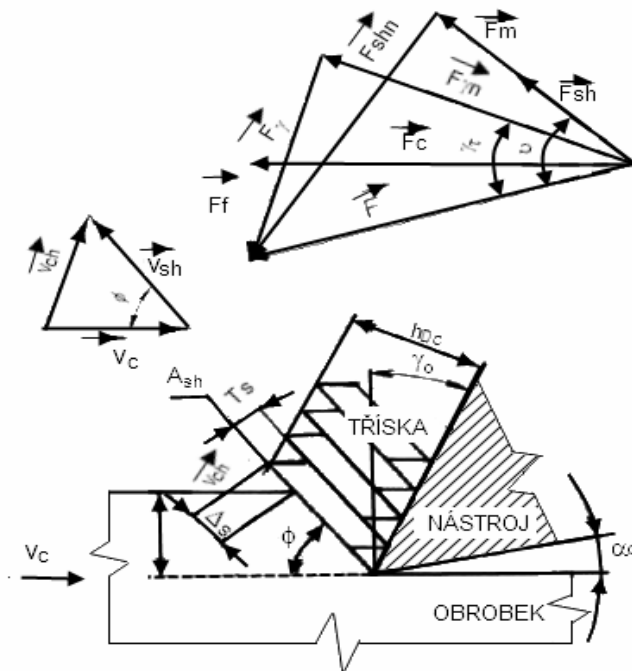
Obr. 2.6 Model tvorby třísky pro HSC obrábění 15
