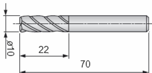
Obr. 4.1 Rozměry fréz
