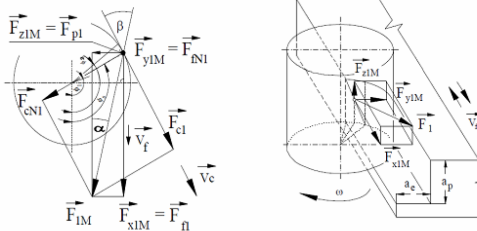
Obr. 2.7 Fyzikální model zatížení řezného nástroje v průběhu obrábění 19
