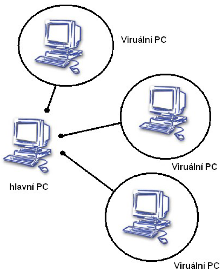
Obr. 13: Virtualizace
