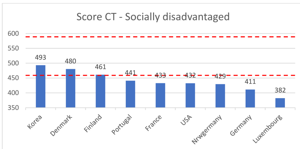
Graf 4 Seřazení skóre IM – sociálně znevýhodnění
