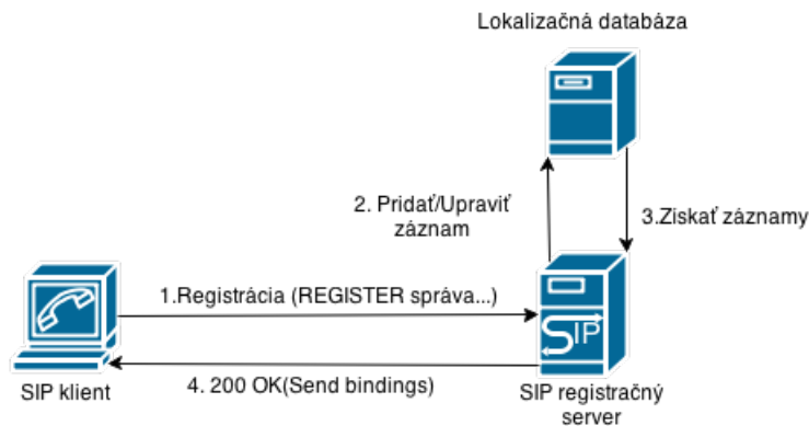
Obrázek 2.1: Schéma registrácie klienta protokolu SIP
