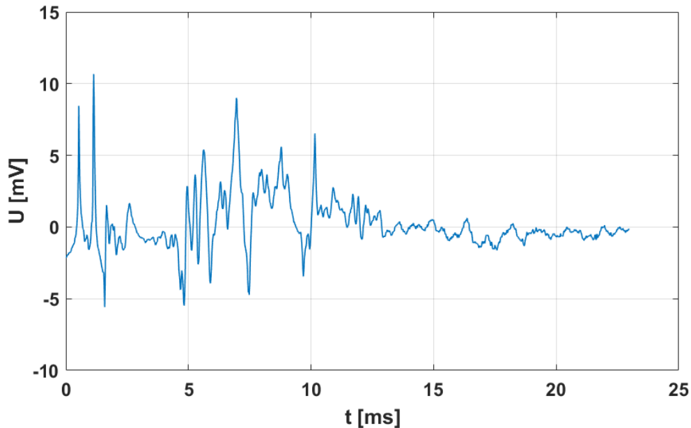
Obrázek 15 Názorný průběh generovaného napětí prvkem DT1-028KL, impuls síly 305 N
