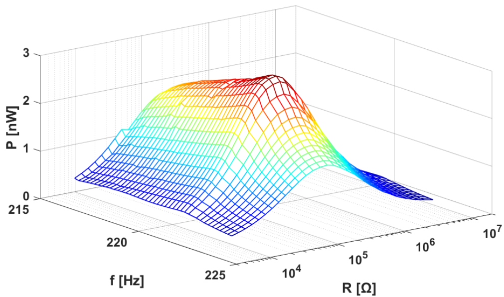
Obrázek B 4 Výkon prvku DT1-028K/L v závislosti na frekvenci a odporovém zatížení, A=4 N_{rms} , f = 215-223 Hz
