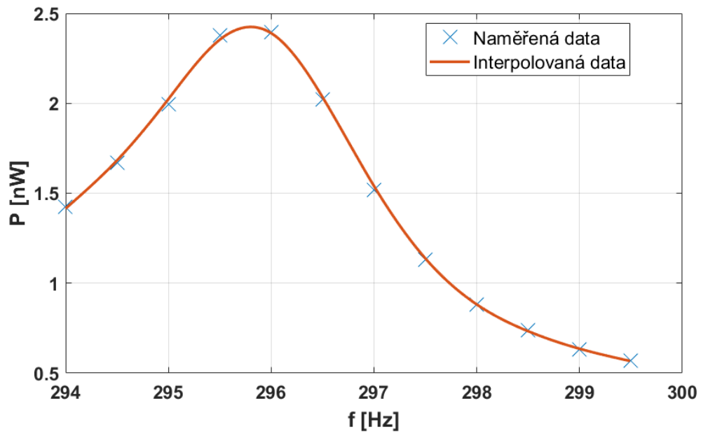
Obrázek B 29 Závislost výkonu prvku DT2-028K na frekvenci při optimálním odporovém zatížení, A=3 N_{rms} , f = 294-300 Hz
