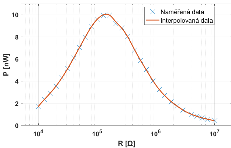
Obrázek B 39 Závislost výkonu prvku LDT2-028K na odporovém zatížení při rezonanční frekvenci, A=4 N_{rms} , f = 295-305 Hz
