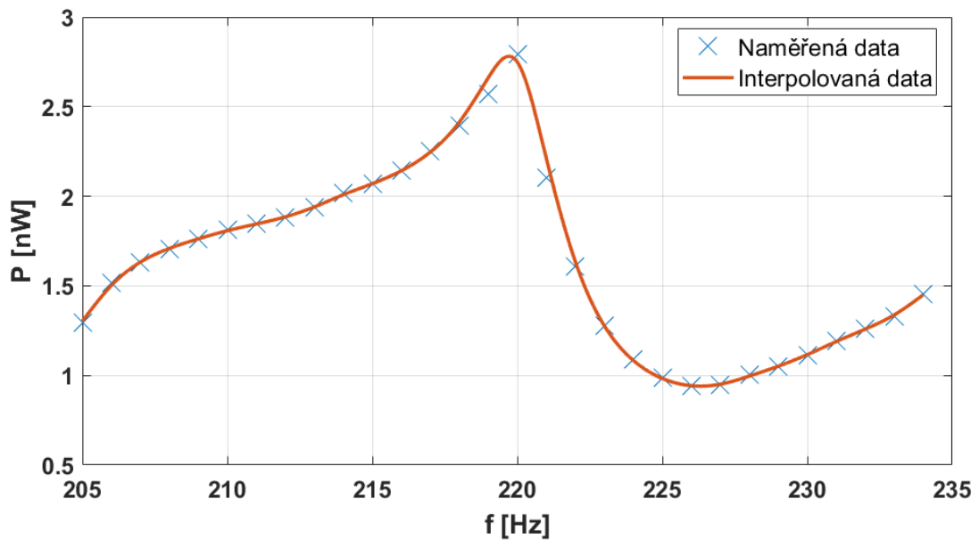
Obrázek B 2 Závislost výkonu prvku DT1-028K/L na frekvenci při optimálním odporovém zatížení, A=4 N_{rms} , f = 205-235 Hz
