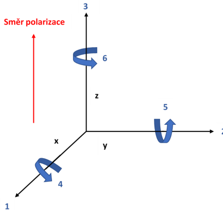
Obrázek 5 Souřadný systém
