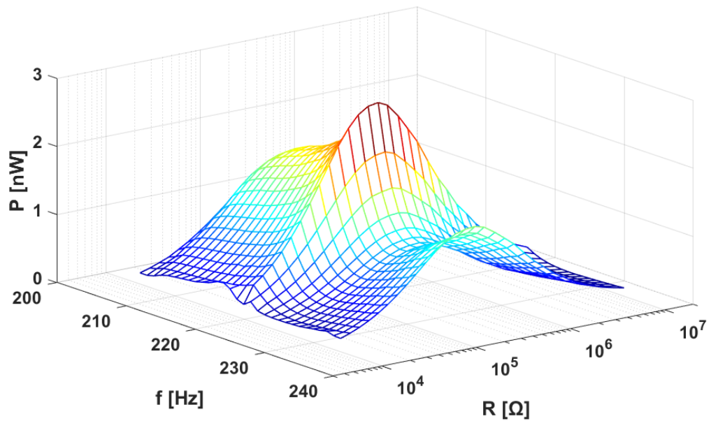
Obrázek B 1 Výkon prvku DT1-028K/L v závislosti na frekvenci a odporovém zatížení, A=4 N_{rms} , f = 205-235 Hz
