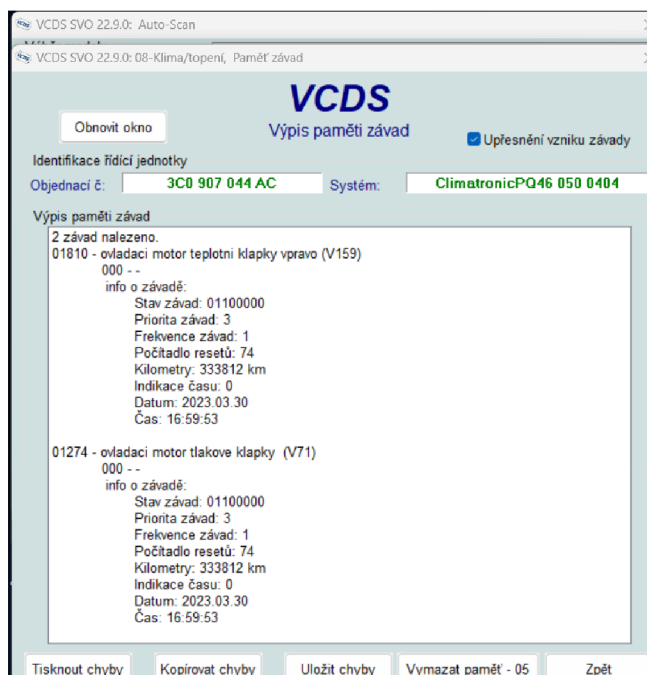
Obrázek 4.3: Závada klimatizace
