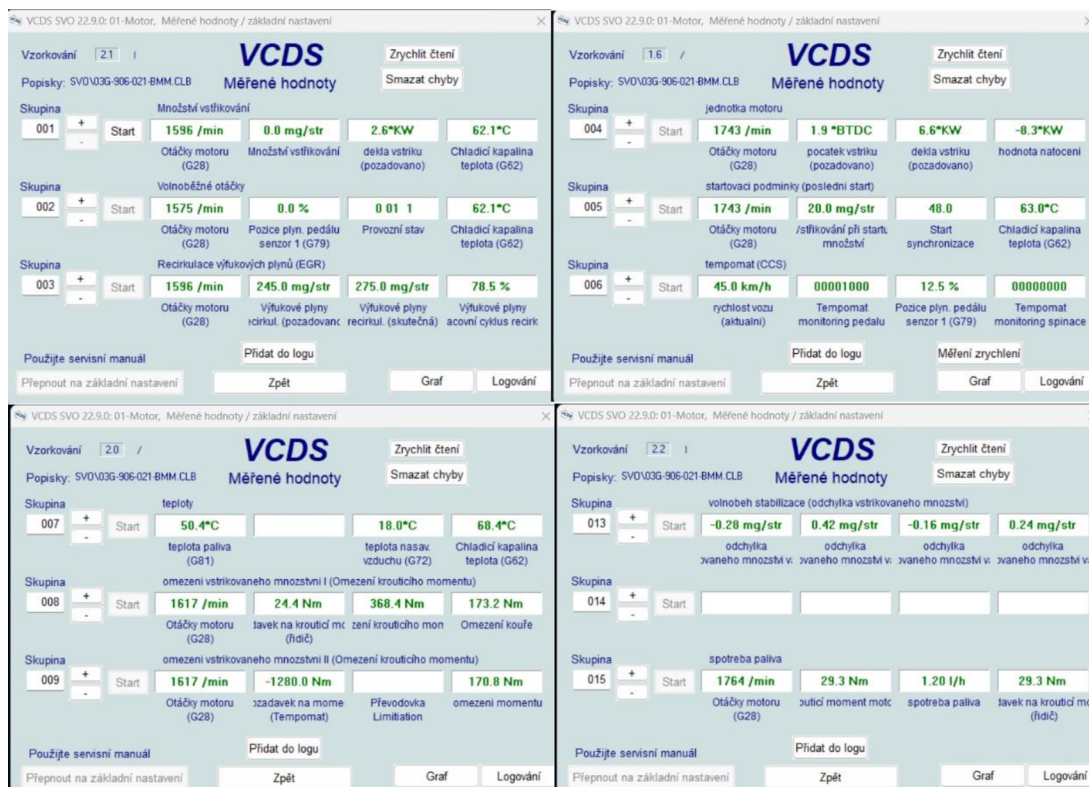
Obrázek 4.4: Měřené hodnoty
