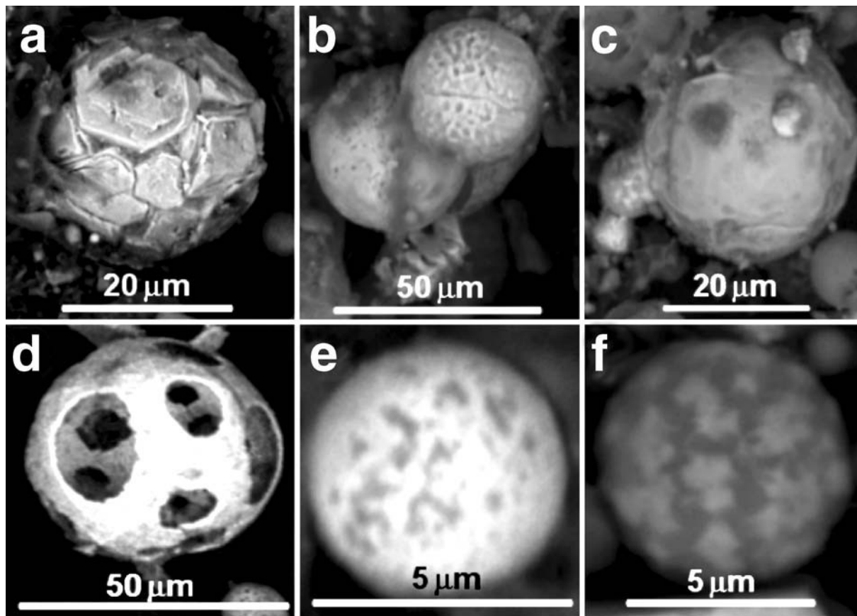
Obrázek 1. Minerální formy obsažené v rhizosféře půd z oblasti jižního Polska (Cabala a Teper, 2007).
