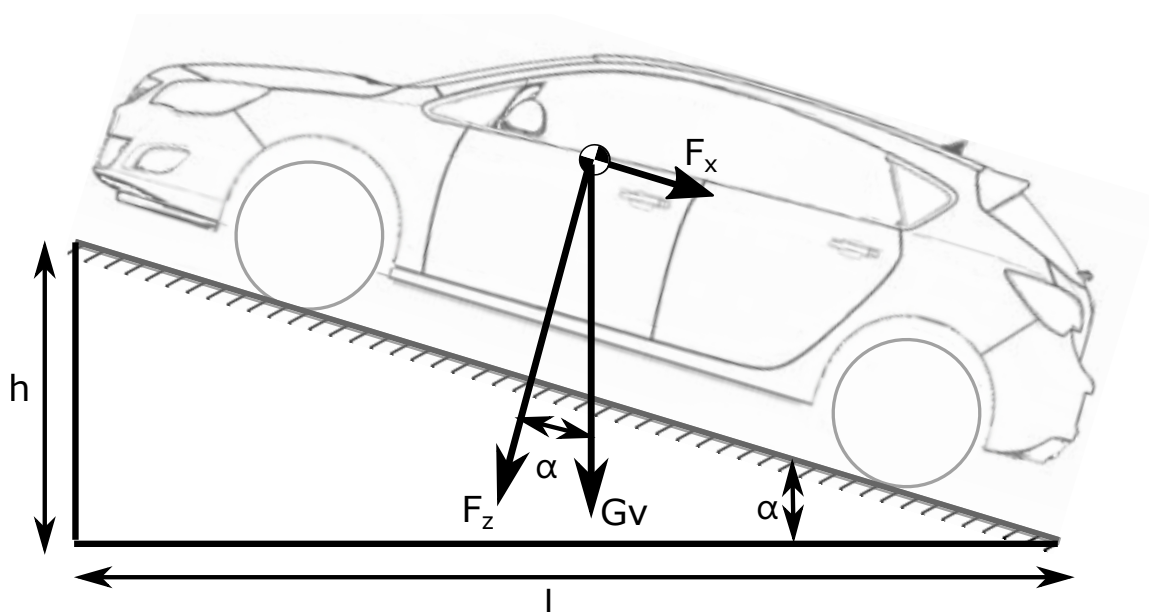
Obrázek 3.9: Fyzikální síly působící na nakloněné rovině, zdroj [25]
