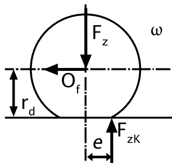
Obrázek 3.10: Fyzikální síly působící na kolo, zdroj [25]
