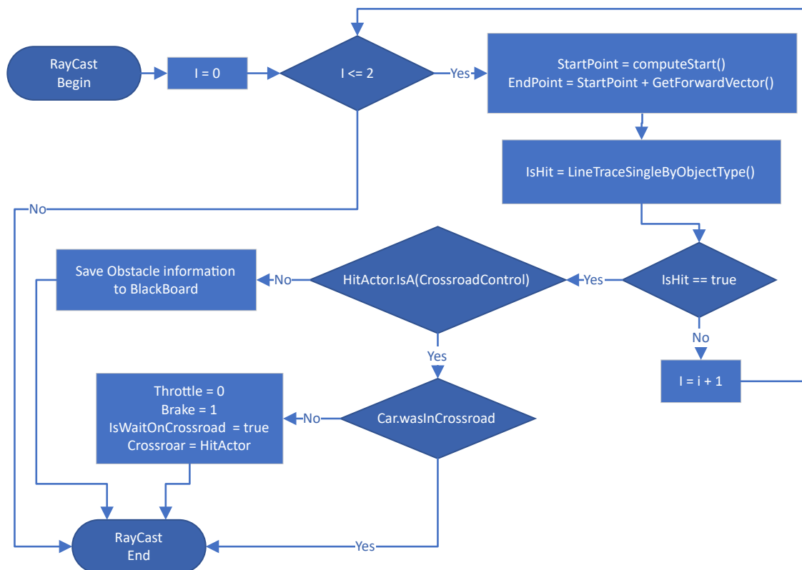
Obrázek 5.10: Vývojový diagram Throttle služby
