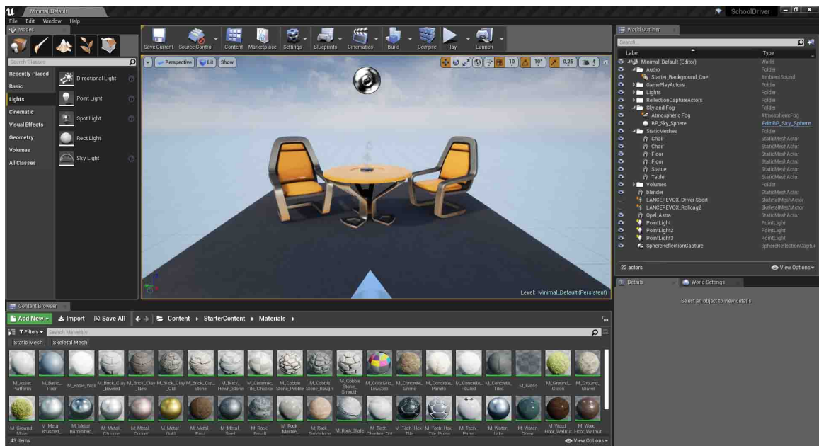
Obrázek 3.5: Unreal Engine
