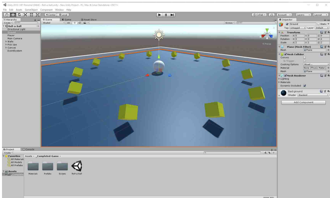
Obrázek 3.3: Unity 3D
