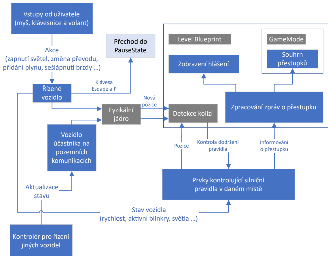
Obrázek 3.15: Architektura simulátoru
