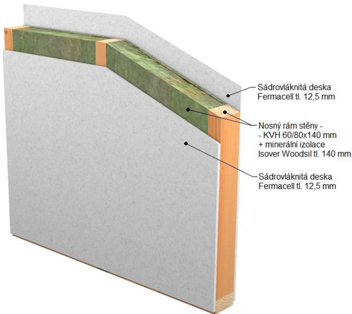
Obrázek 33 - Skladba W7 – vnitřní příčka tloušťky 165 mm (autor práce, 2024)
