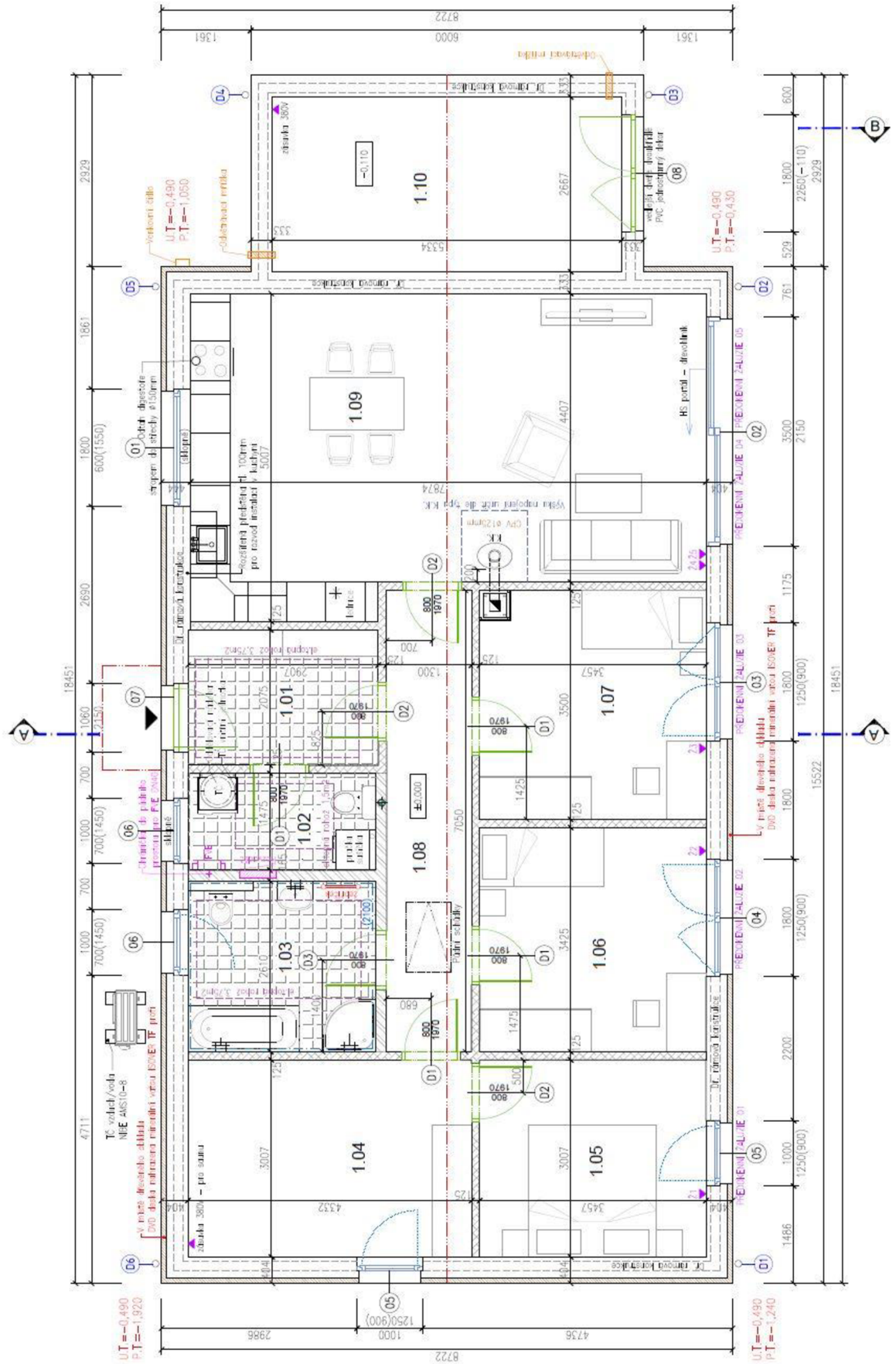
Obrázek 20 - Půdorys objektu ze zvoleného projektu – použito se souhlasem autora dokumentace pro stavební povolení (Viktor Beníšek, 2022)
