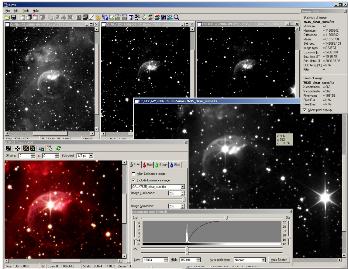
Obrázek 13: Program SIPS [7]
