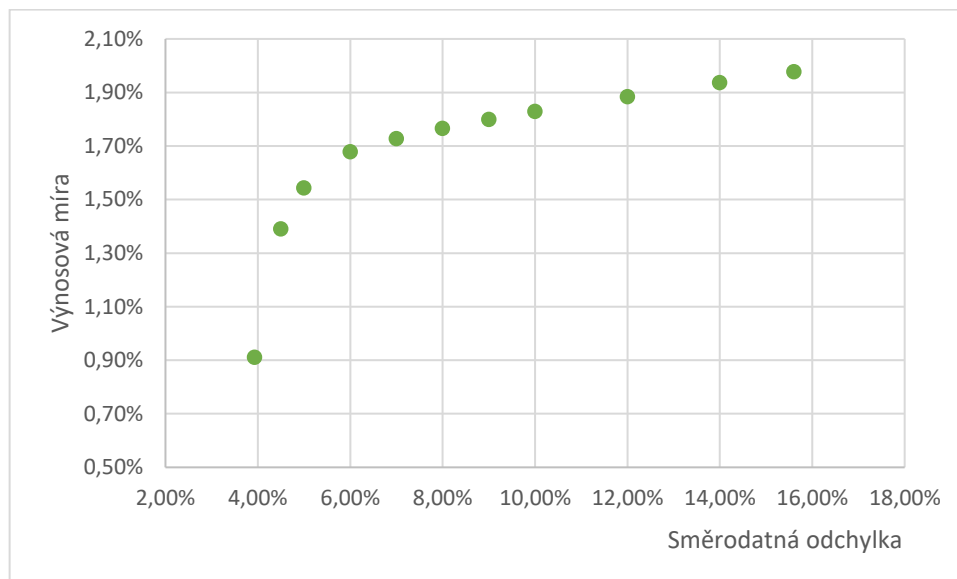
Graf 4 Efektivní hranice – Americké portfolio
