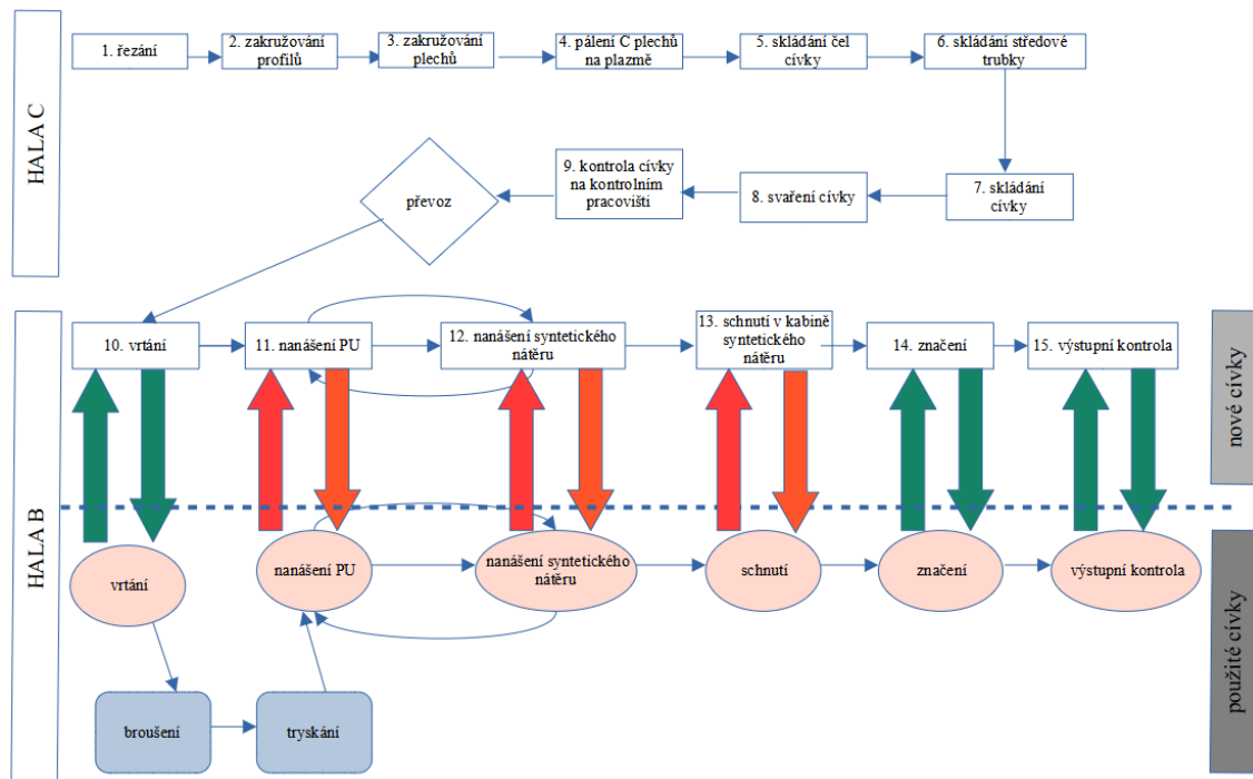
Obr. 3.12 Schéma výrobního diagramu pracovních činností
