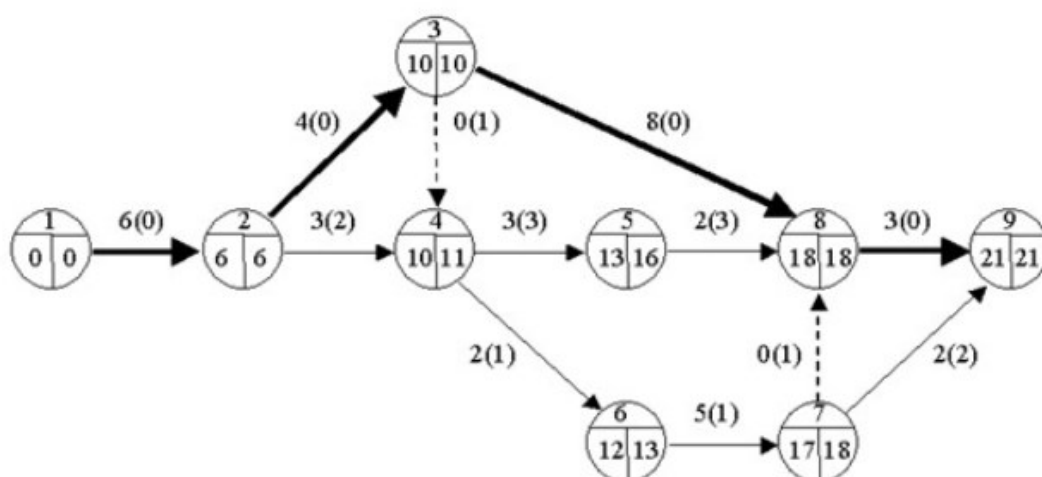
Obr. 2.6 Výpočet nejpозději přípustných konců a celkových časových rezerv
