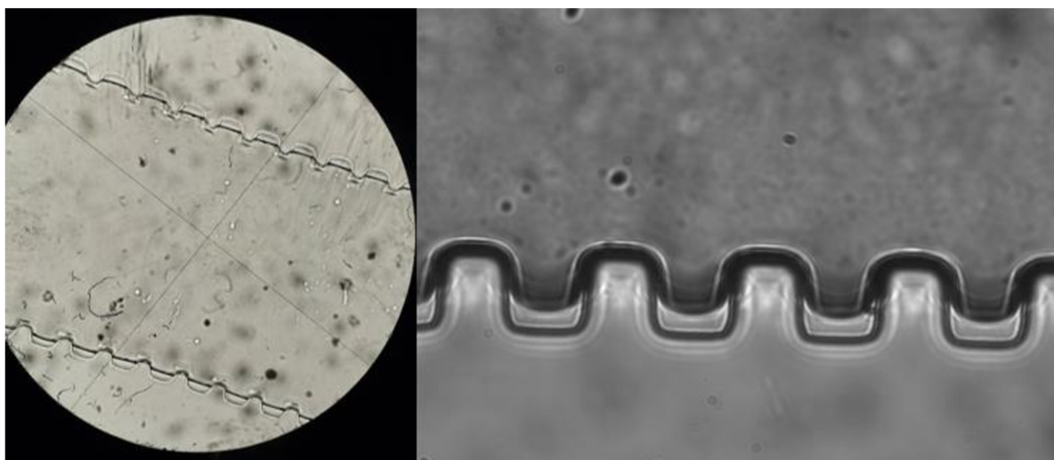
Obrázek 14: Hexadekan zablokovaný uvnitř kanálku
