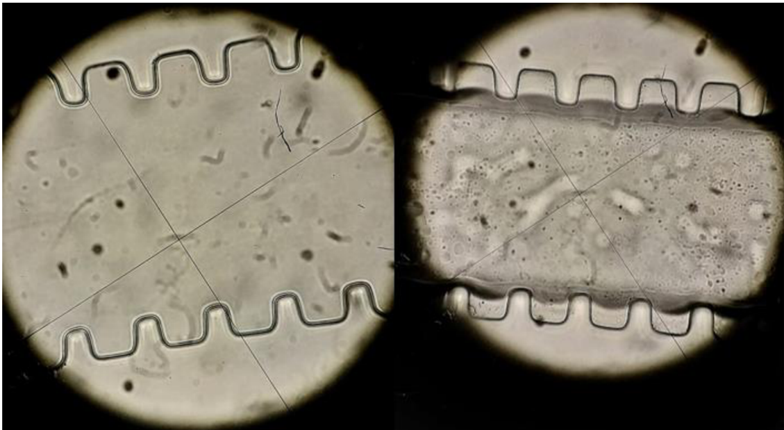
Obrázek 10: Kanálky o šířce 100 µm (vlevo – naplněný roztokem PBS; vpravo – naplněný roztokem lecitinu v hexadekanu)
