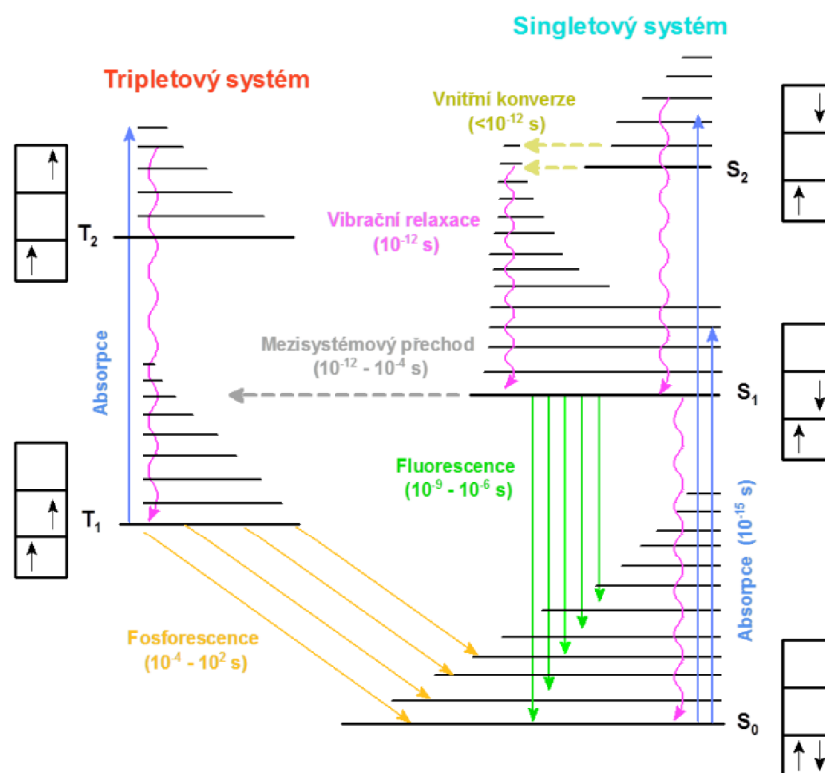
Obrázek 5: Jablonskiho diagram [16]
