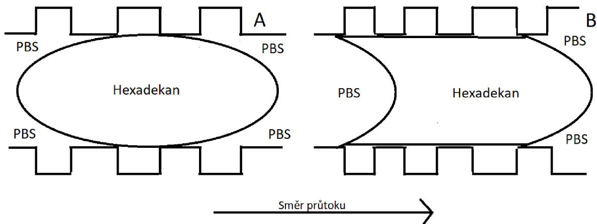
Obrázek 12: A – normální (konkávní) tvar hexadekanu; B – konvexní tvar hexadekanu (tvary se vztahují na první rozhraní ve směru průtoku)
