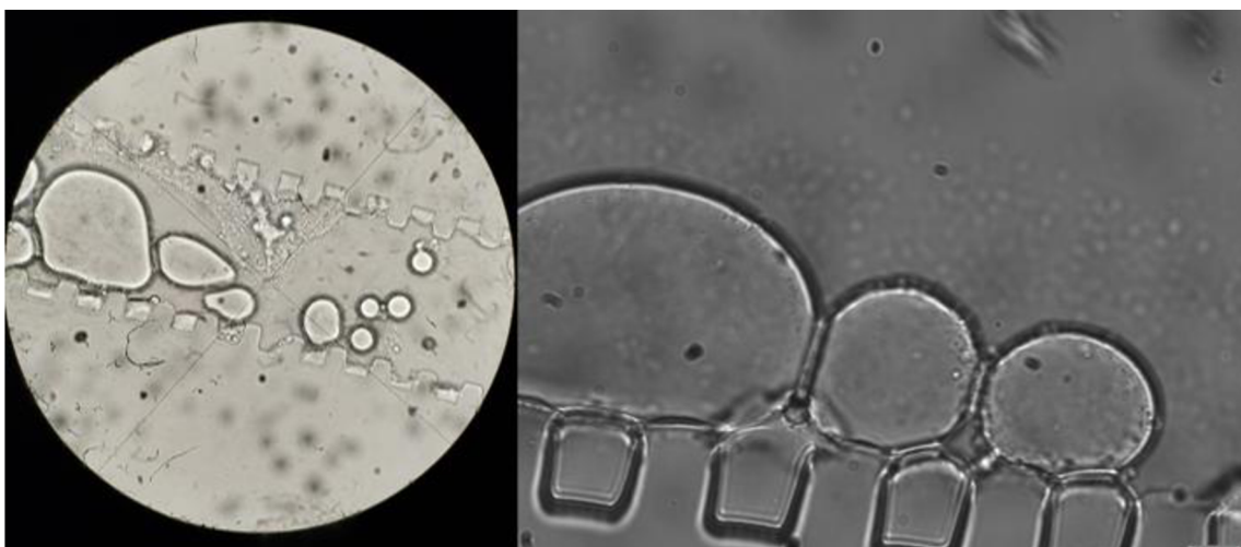
Obrázek 13: Části hexadekanu v kanálku
