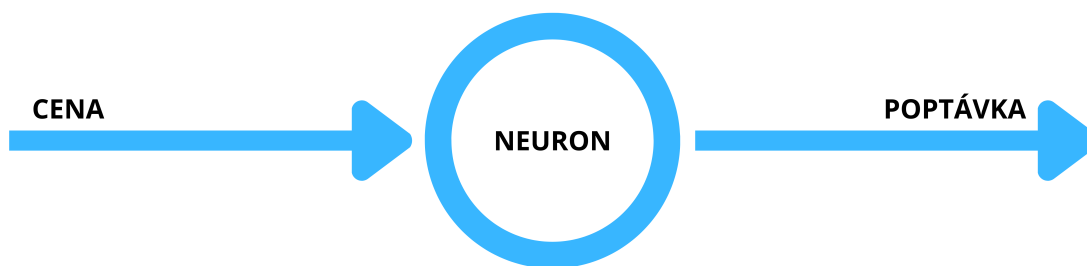
Obrázek 1.1: Neuron
