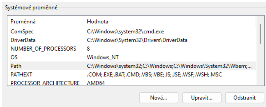
Obrázek 4.2: Systémové proměnné
