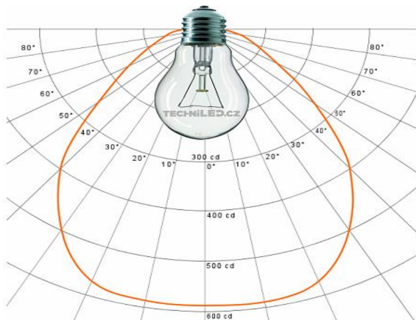
Obrázek 4 Diagram svítivosti
