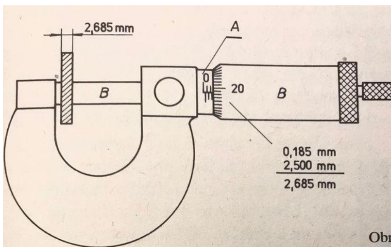
Obrázek 10 Mikrometrický šroub
