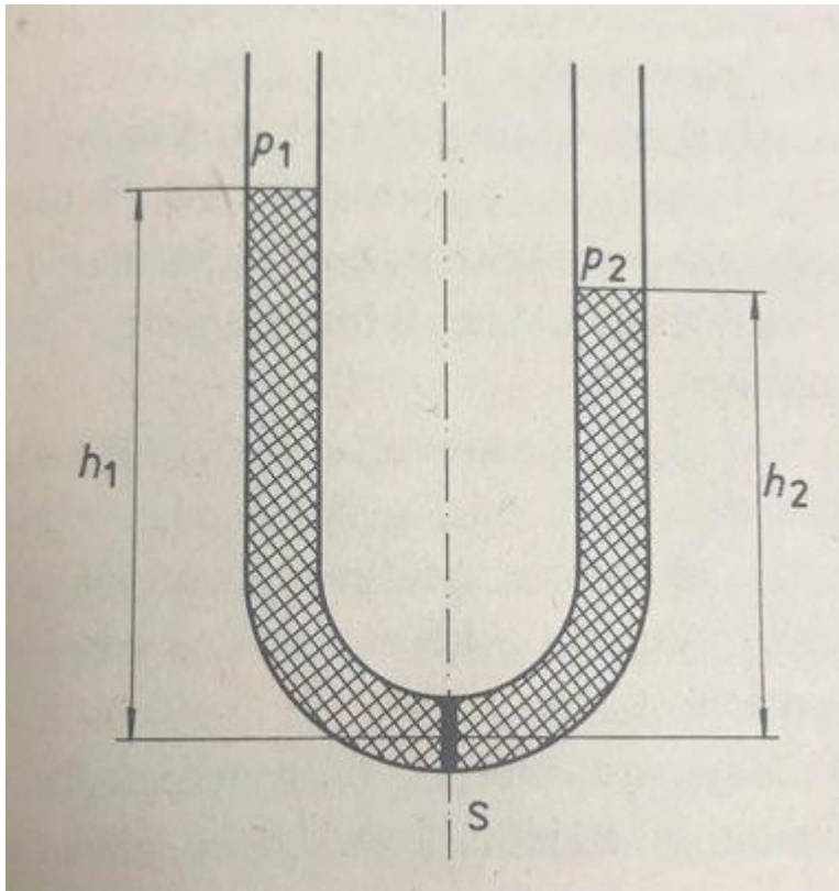
Obrázek 11 U-manometr
