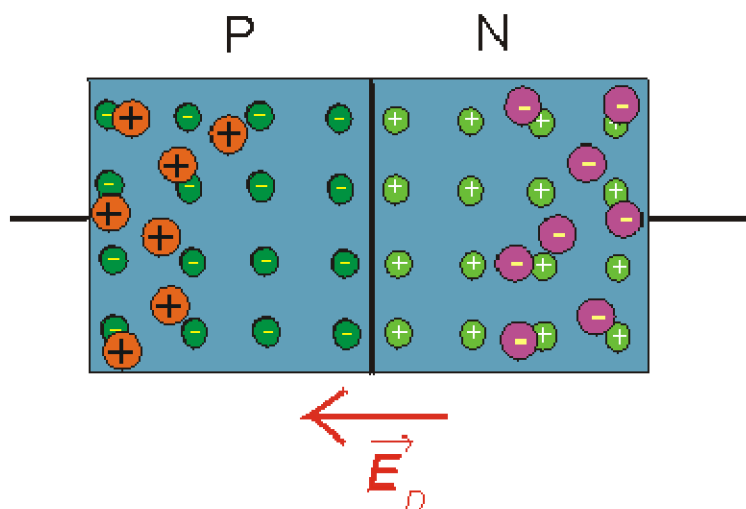
Obr. 5-4 PN přechod v rovnovážném stavu
