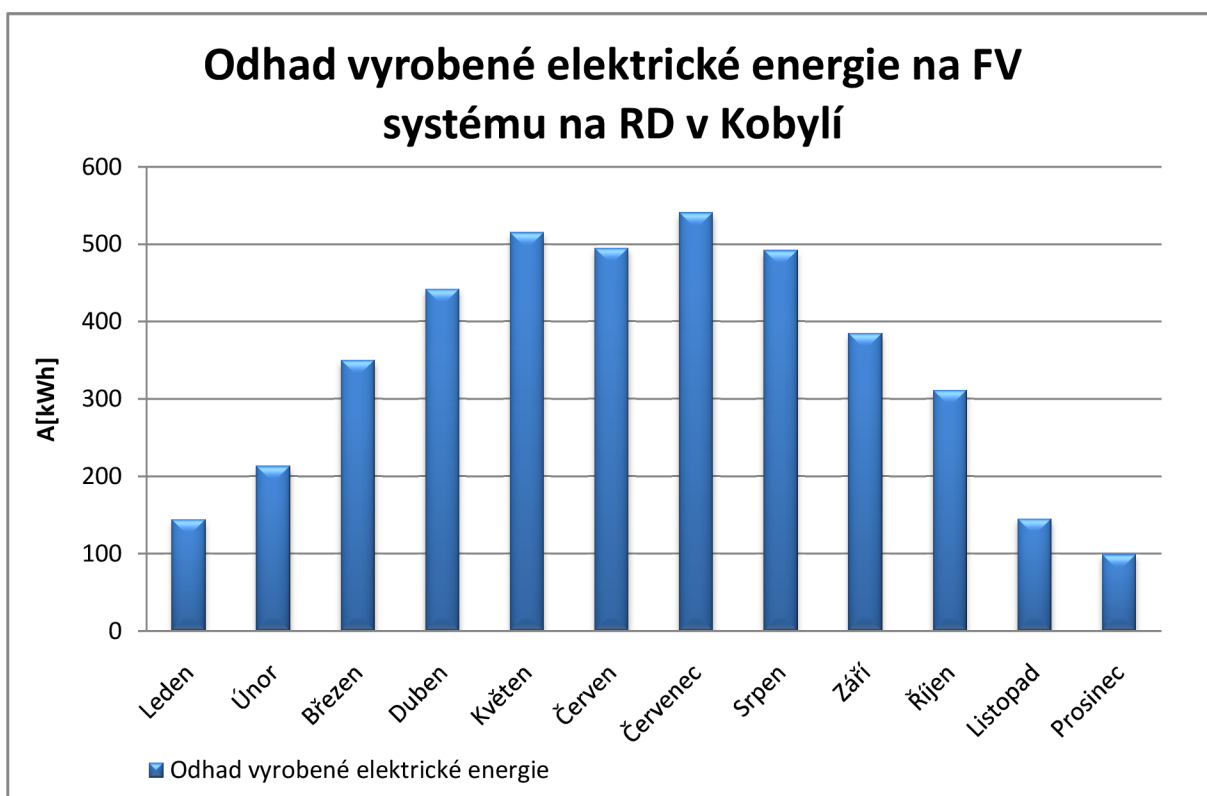
Obr. 10-1 Odhad průměrného množství vyrobené el. energie
