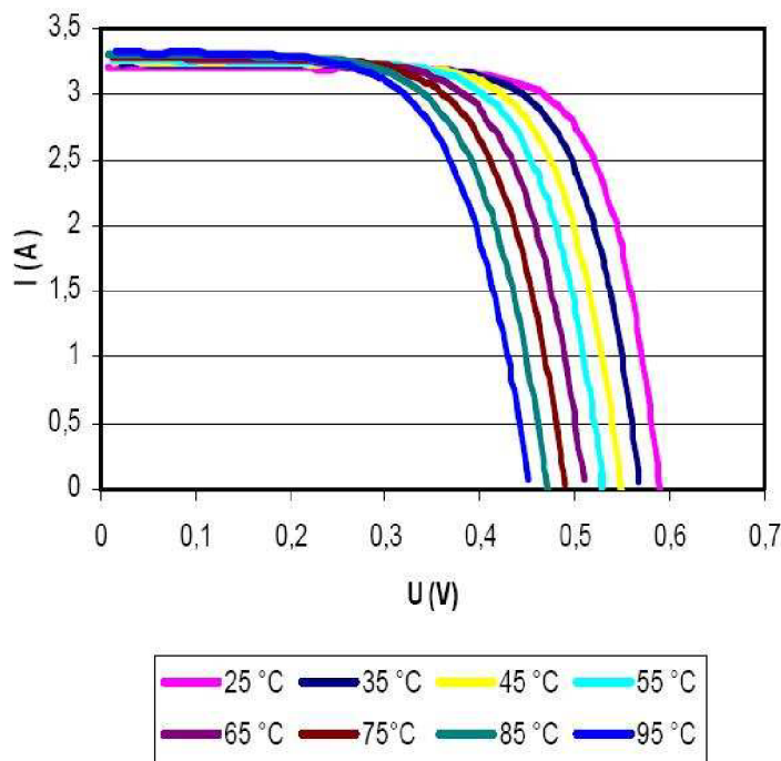
Obr. 6-5 Vliv teploty V-A charakteristiky fotovoltaických článků při I = 1000 \text{ Wm}^{-2}
