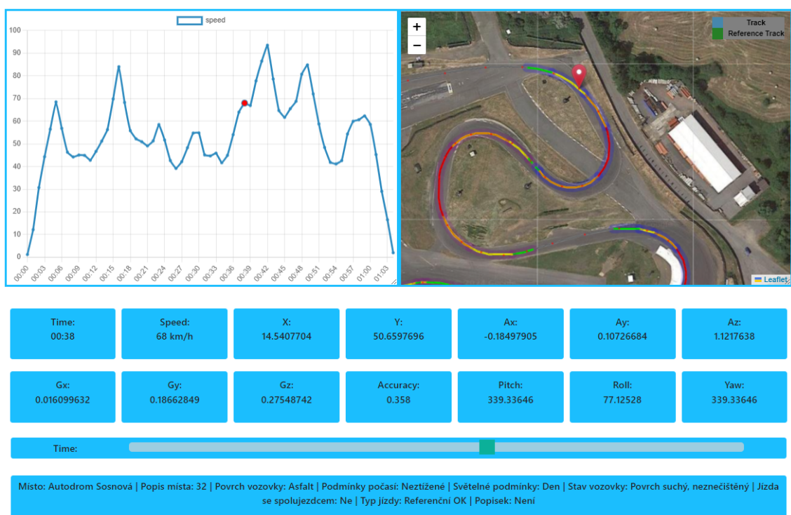
Obrázek 4.5: Vzhled hotové stránky pro vizualizaci dat
