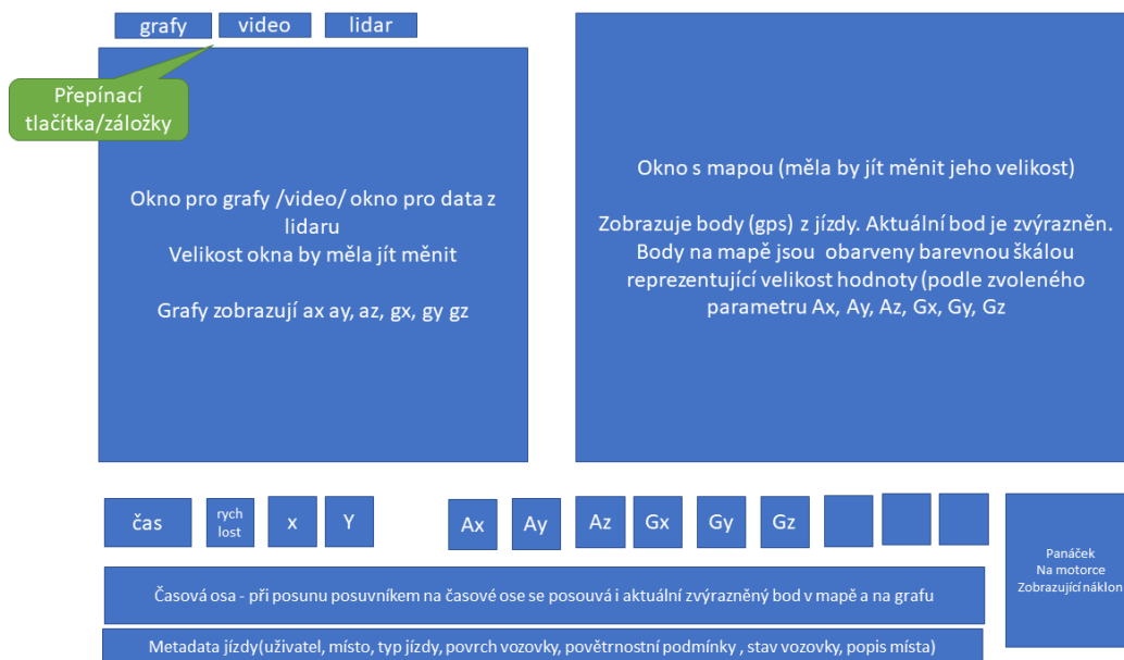
Obrázek 4.1: Vizualizace požadavku na UI
