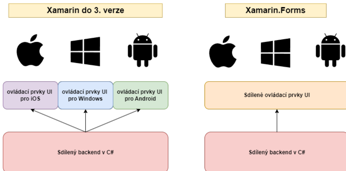
Obrázek 2.2: Architektura Xamarinu
