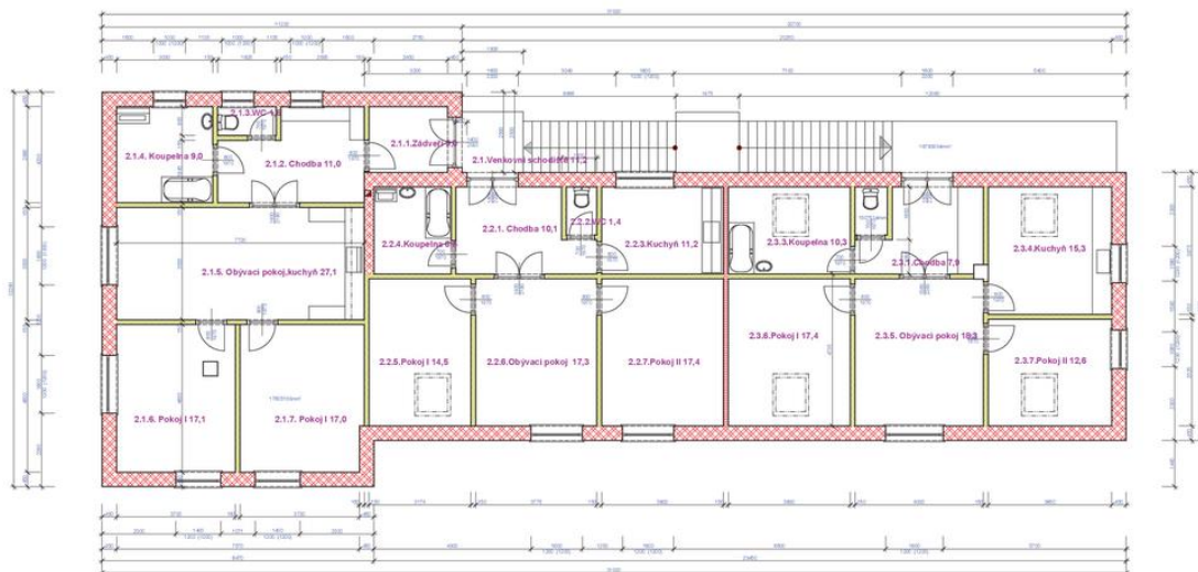
Obrázek č. 5 – Dispozice bytů [33]
