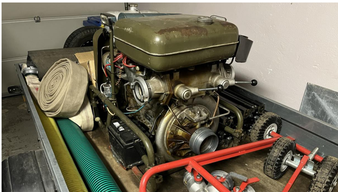
Obrázek 2: Příklad přenosné motorové stříkačky
