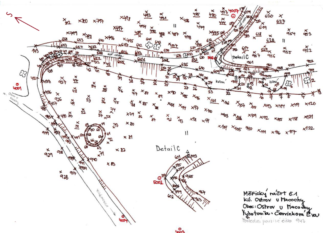
Obrázek 15: Měřický náčrt č.1
