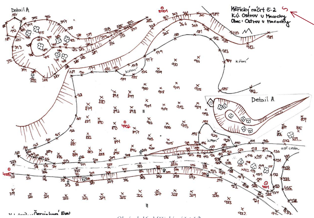
Obrázek 16: Měřický náčrt č.2
