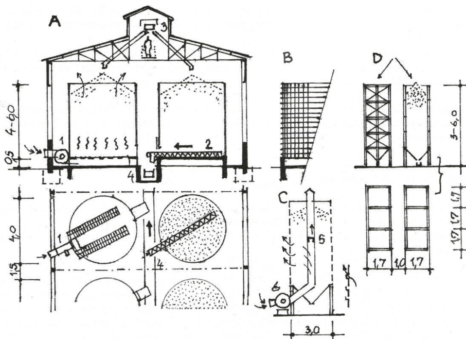
Obrázek 10: Kombinovaný sklad obilí, A – příklad celkové sestavy, B – schéma síla z ocelových prutů vyložených PVC folií, C – plechové dosoušecí silo, D – stavebnicová síla z ocelové příhradoviny, vyložené pogumovanou plachtovinou, 1 – vzduchové potrubí s ventilátorem, 2 – vyprázdňení šnekem a vyfoukání, 3 – plnicí pás se shrnovacím zařízením, 4 – vyprázdňovací pás, 5 – posuvná zátka (nutí vzduch prostoupit obilím a perforovanou stěnou), 6 – teplovzdušný ventilátor, (Sýkora, 2014)
