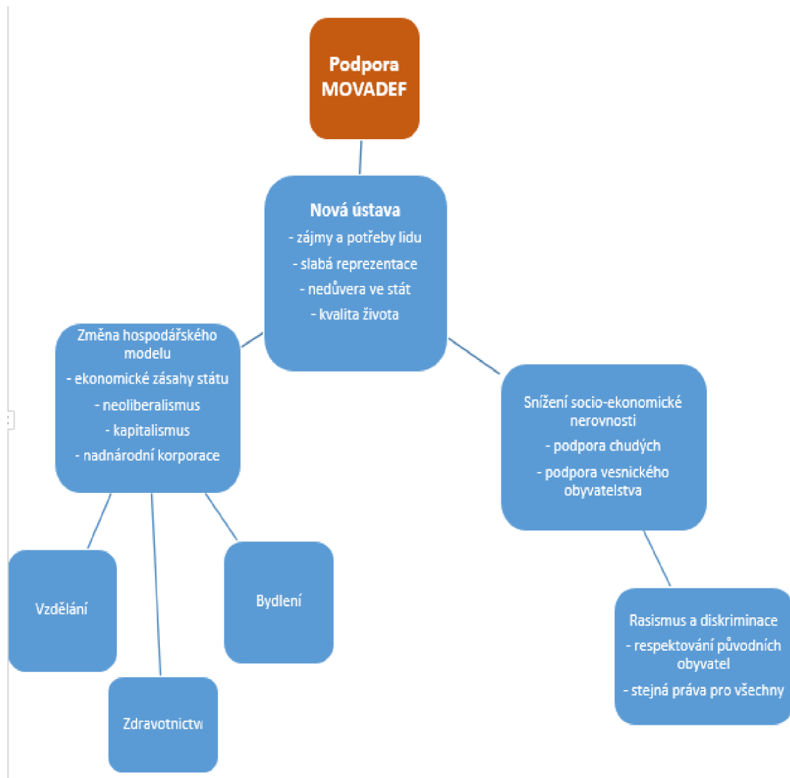
Obrázek 2 - Selektivní kódování
