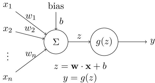
Obrázek 3.1: Ukázka umělého neuronu s n vstupy x , váhami w a aktivační funkcí g .
