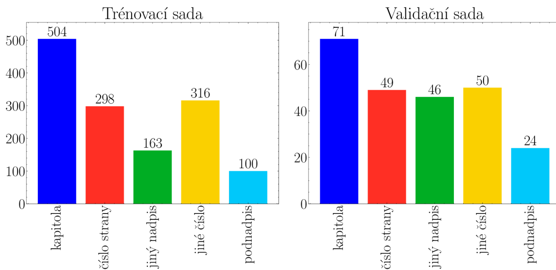
Obrázek 4.2: Rozložení tříd datové sady knih. Jedná se počet o ground truth anotací s metadaty dané třídy.
