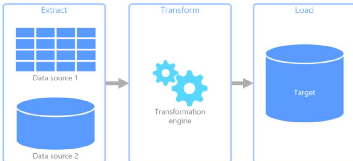
Obrázek 4: ETL schéma [25]
