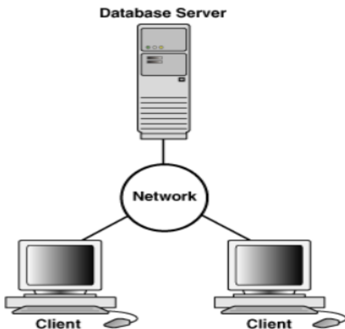
Obrázek 2: CLIENT/SERVER schéma [7]
