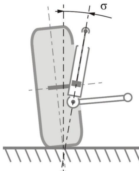
Obr. 20 Úhel příklonu rejdrové osy [33]
