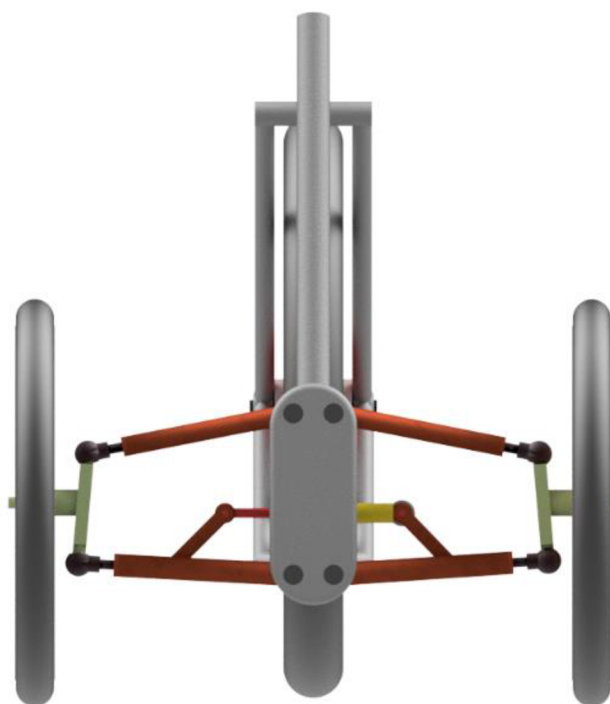
Obr. 28 pohled zepředu
