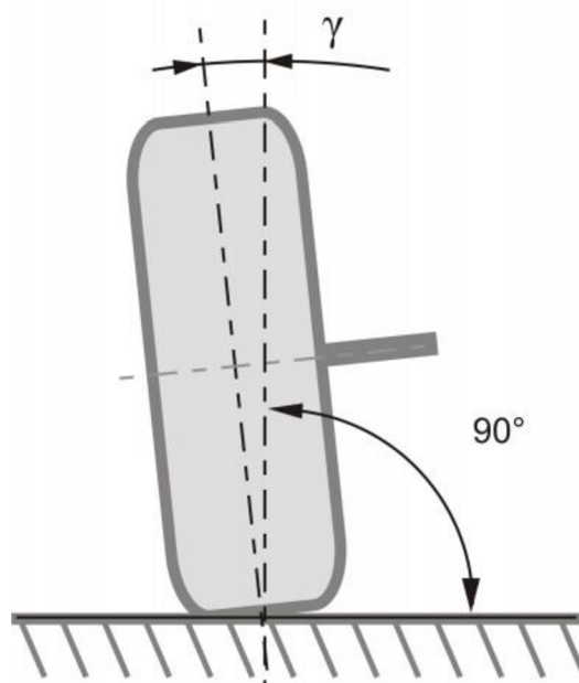
Obr. 18 Odklon kola [32]
