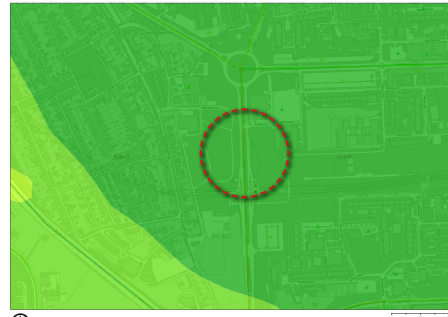
Obrázek č. 32: Kvalita ovzduší
