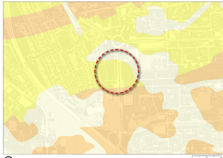
Obrázek č. 30: Geologické ukazatele
