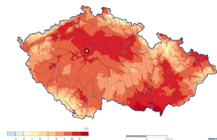
Průměrná roční teplota vzduchu v roce 2022
