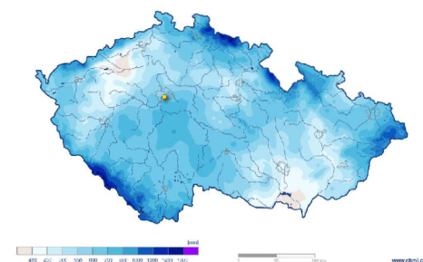
Úhrn srážek v roce 2022
