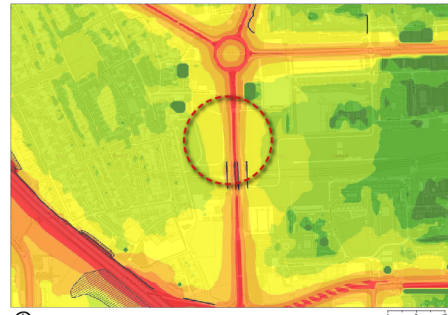
Obrázek č. 33: Hluková mapa
