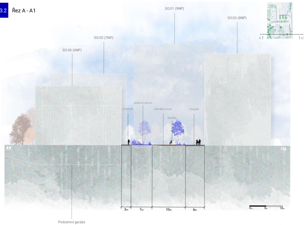
Obrázek č. 71: Řez A-A1 Zdroj: autor práce
