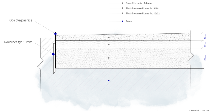
Obrázek č. 101: Technický detail C - Mlatová cesta Zdroj: autor práce
