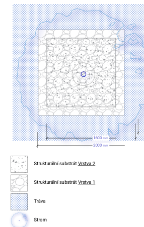
Obrázek č. 95. Technický detail B - strukturální substrát Zdroj: autor práce
