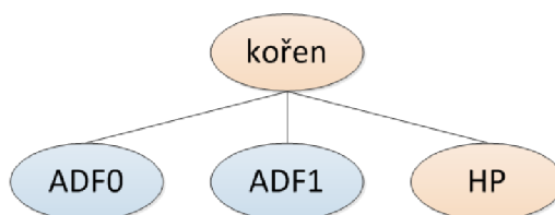
Obrázek 2.4: Schéma stromu s automaticky definovanými funkcemi.
