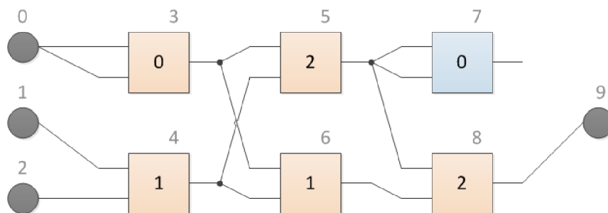
Obrázek 3.1: CGP - příklad kandidátního obvodu. Uzel č. 7 není v fenotypu využit.
