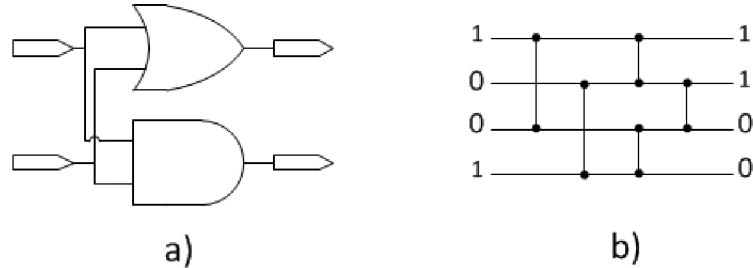
Obrázek 7.5: Řadicí síť: a) schéma komparátoru b) schéma 4-bitové řadicí sítě. Svislé čáry značí připojení komparátorů.
