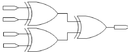
Obrázek 7.4: Schéma zapojení funkcí XOR ve větším modulu. V implementaci byl XOR sestaven z hradel AND, OR a NAND.
