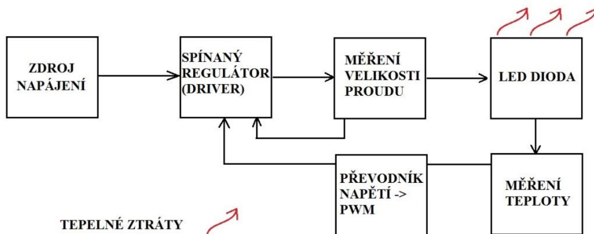
Obr. 16: Blokový náčrt spínané regulace proudu řízené teplotou
