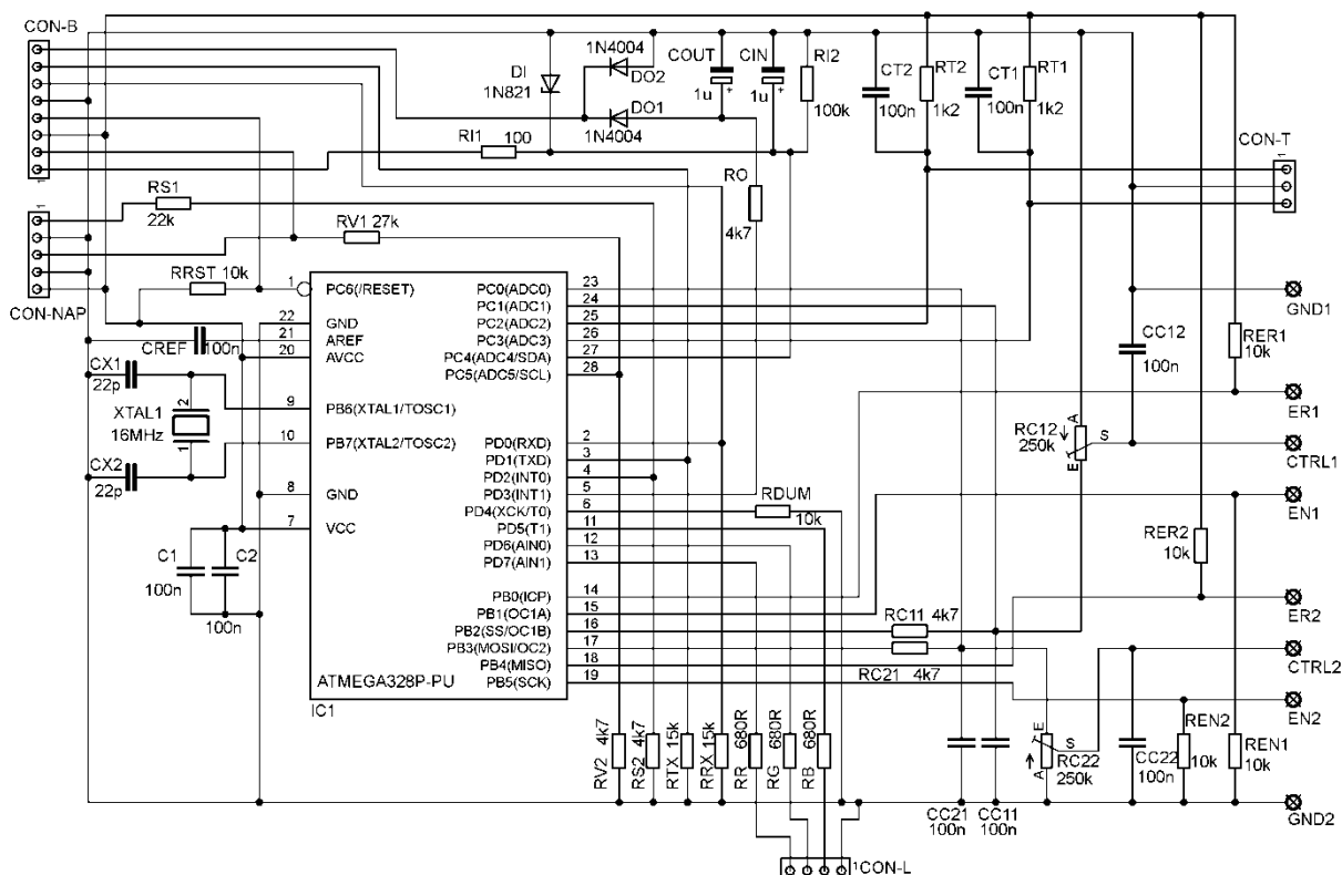
Obr. 30: Schéma zapojení ovládací části pro návrh DPS v programu Eagle
