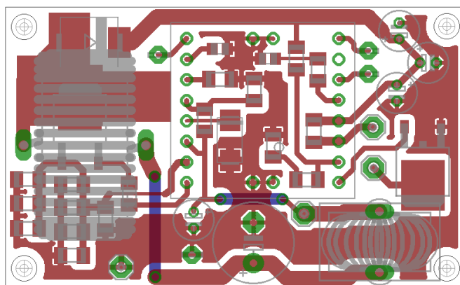
Obr. 29: Obrazec spojů navržené DPS driveru s obrysy součástek
