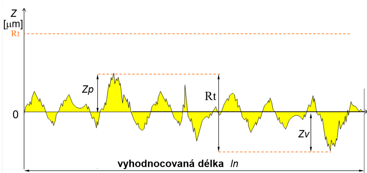
Obr. 11 Znáornění parametru R_t [3]
