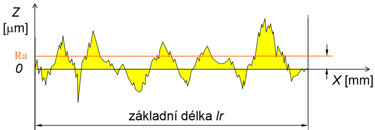
Obr. 10 Znáornění parametru Ra [3]
