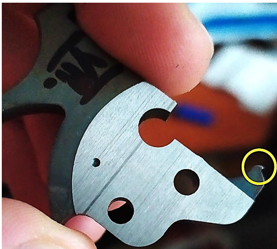
Obr. 23 Funkční plocha kohoutu a ostrý zobáček
