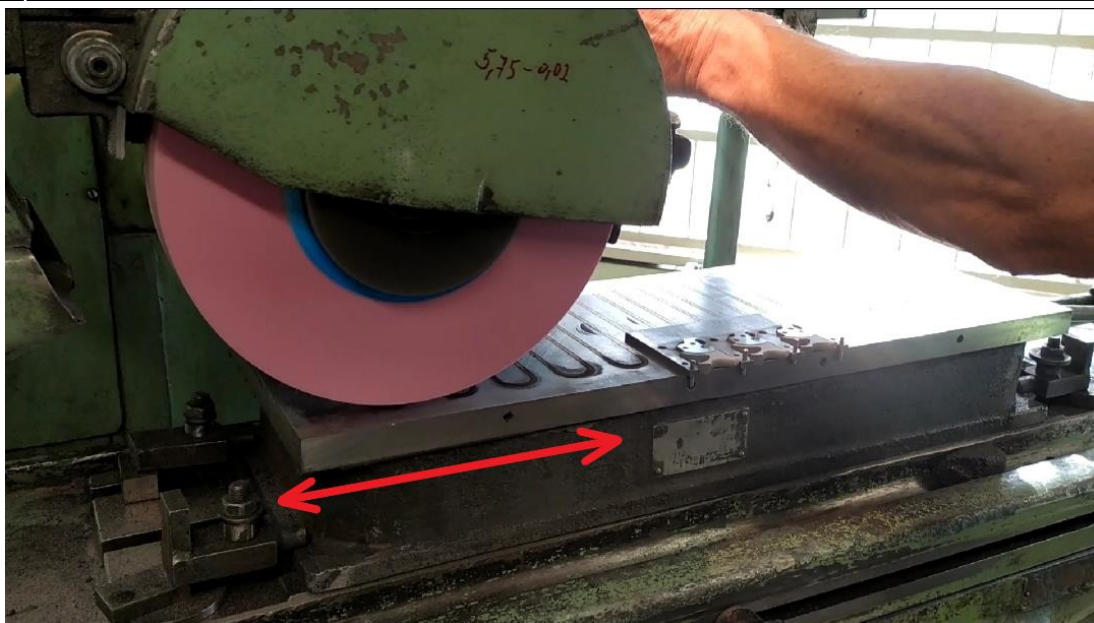
Obr. 24 Rovinná bruska během broušení kohoutů
