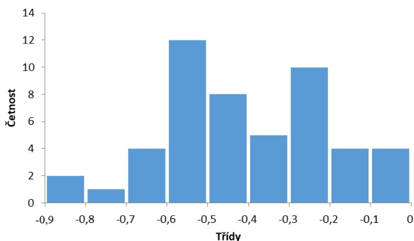
Obr. 44 Parametr Rsk – broušený povrch, nový kotouč
