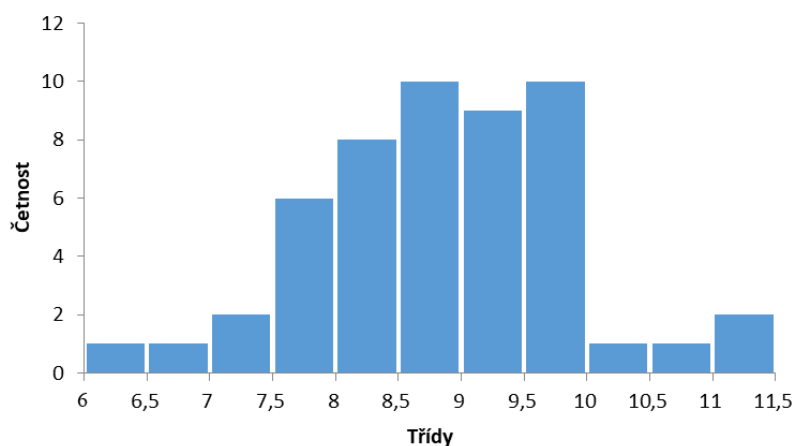
Obr. 53 Parametr Sz – broušený povrch, nový kotouč
