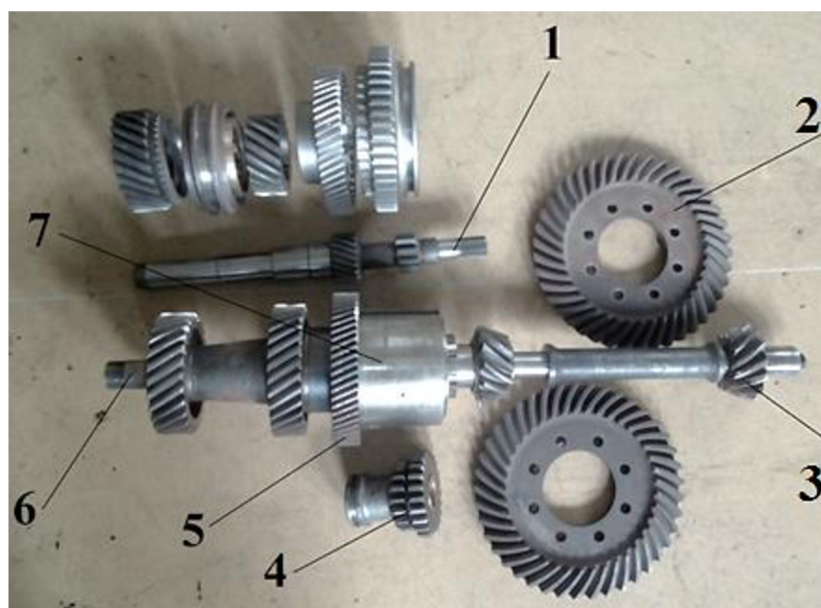
Obr. 6-11 Jednotlivé části převodové skříně
