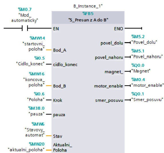
Obr. 4.4: Volání funkčního bloku “5_Presun z A do B”
