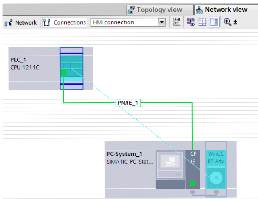
Obr. C.3: Vytvoření spojení PLC a HMI
