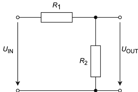
Obr. 1.1: Schéma L-článku
