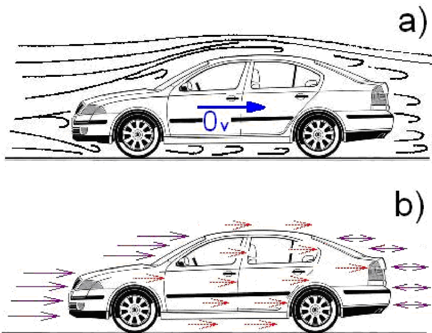
Obr. 1.17 a) Průběh proudnic vozidla obtékaného vzduchem, b) Vznik vzdušného odporu z tlakových sil (plné fialové šipky) a třecích sil (čárkované červené šipky)
