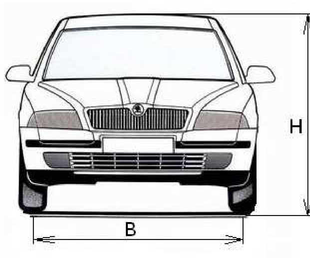
Obr. 1.23 Obrys vozidla [14]
