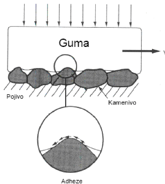
Obr. 1.7 Styk pneumatiky s vozovkou [20]
