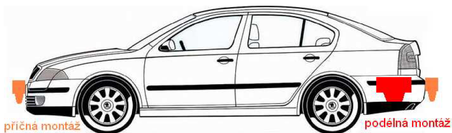
Obr. 3.3 Pozice uchycení měřícího zařízení Correvit na vozidle Pozn.: vlastní úprava podle [18]
