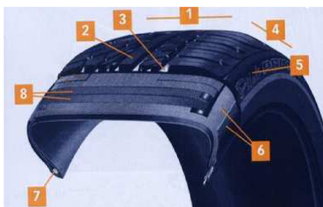
Obr. 1.2 Konstrukční prvky pneumatiky [8]
