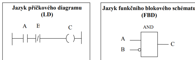
Obrázek 2-5 Logická funkce AND ve čtyřech základních jazycích [14]
