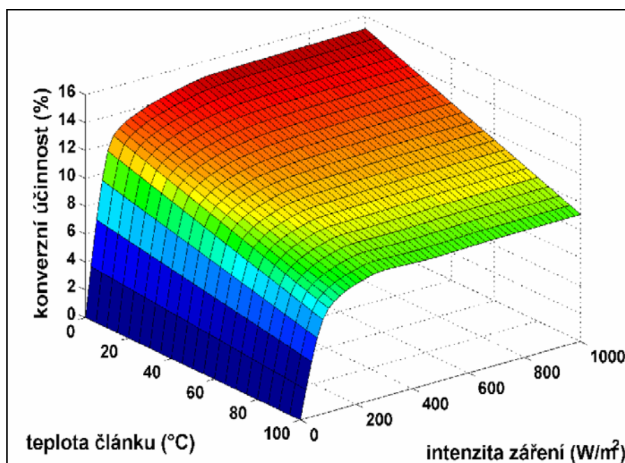
Graf 2 Křivka účinnosti článku, zdroj [4]
